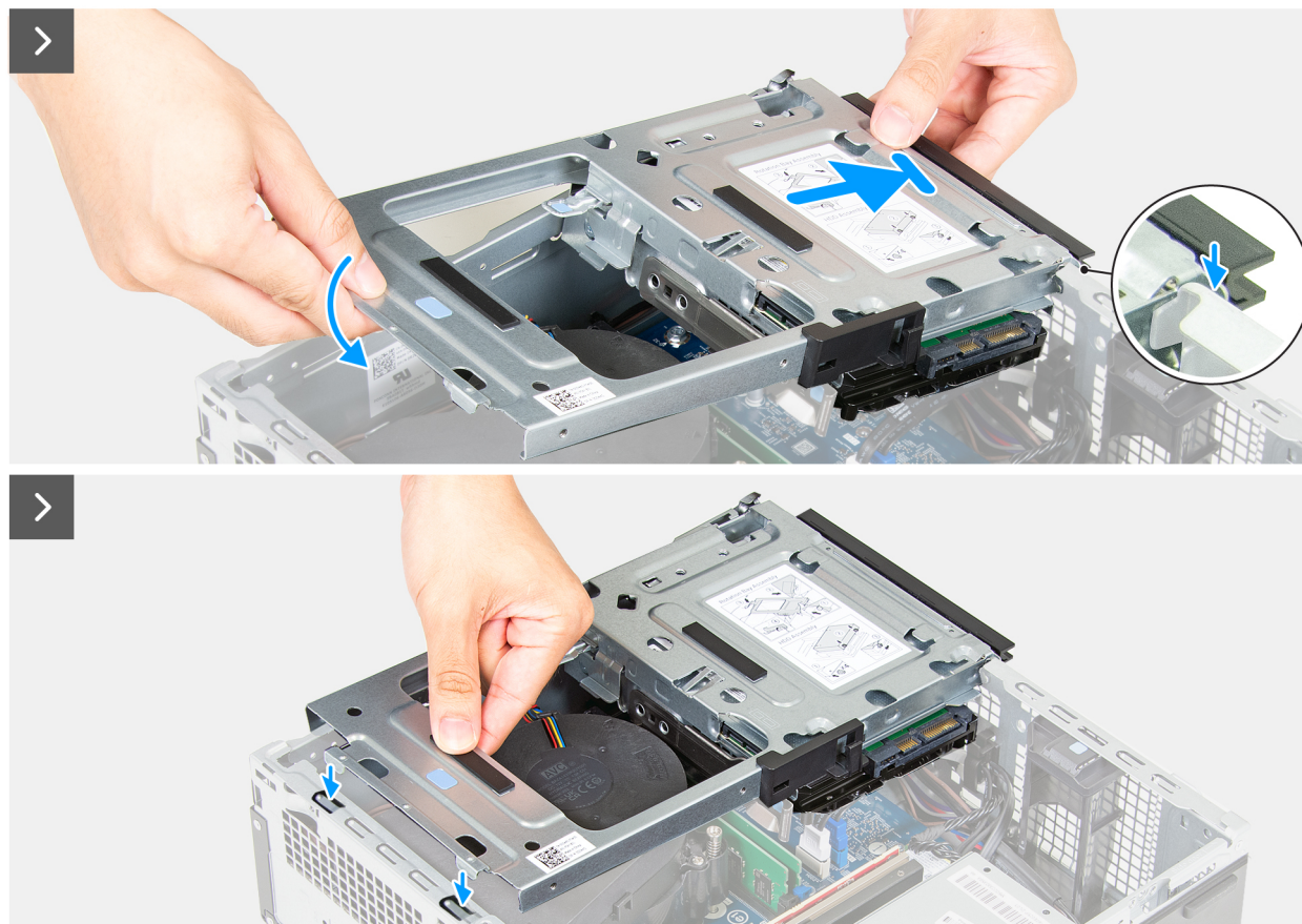
Ilustración 37. Instalación del compartimiento de la unidad
