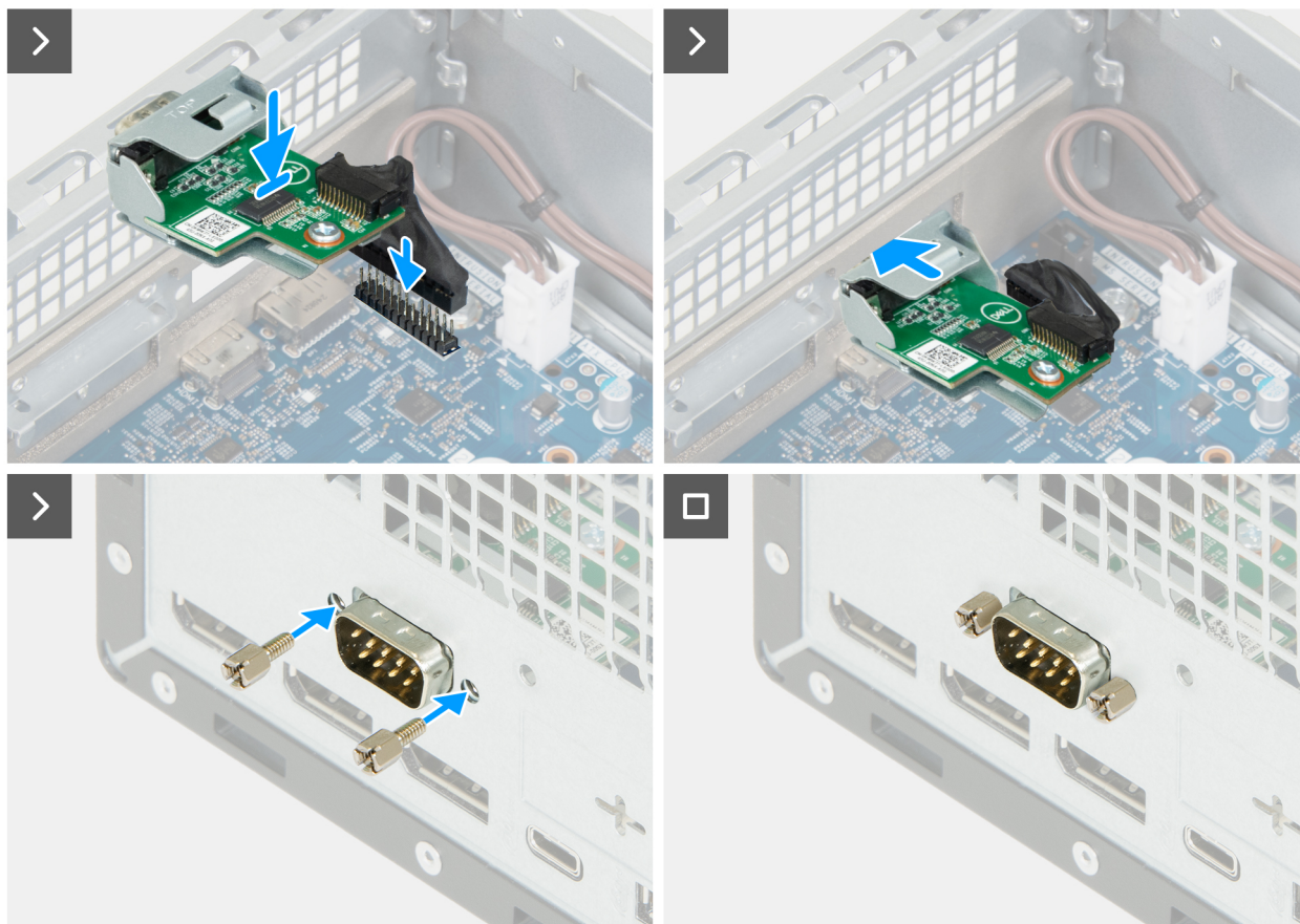
Ilustración 58. Cómo instalar el módulo de puerto serial
