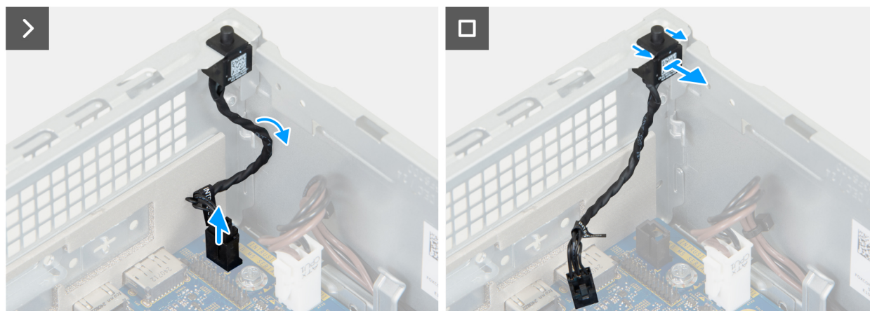
Ilustración 41. Extracción del switch de intrusiones
