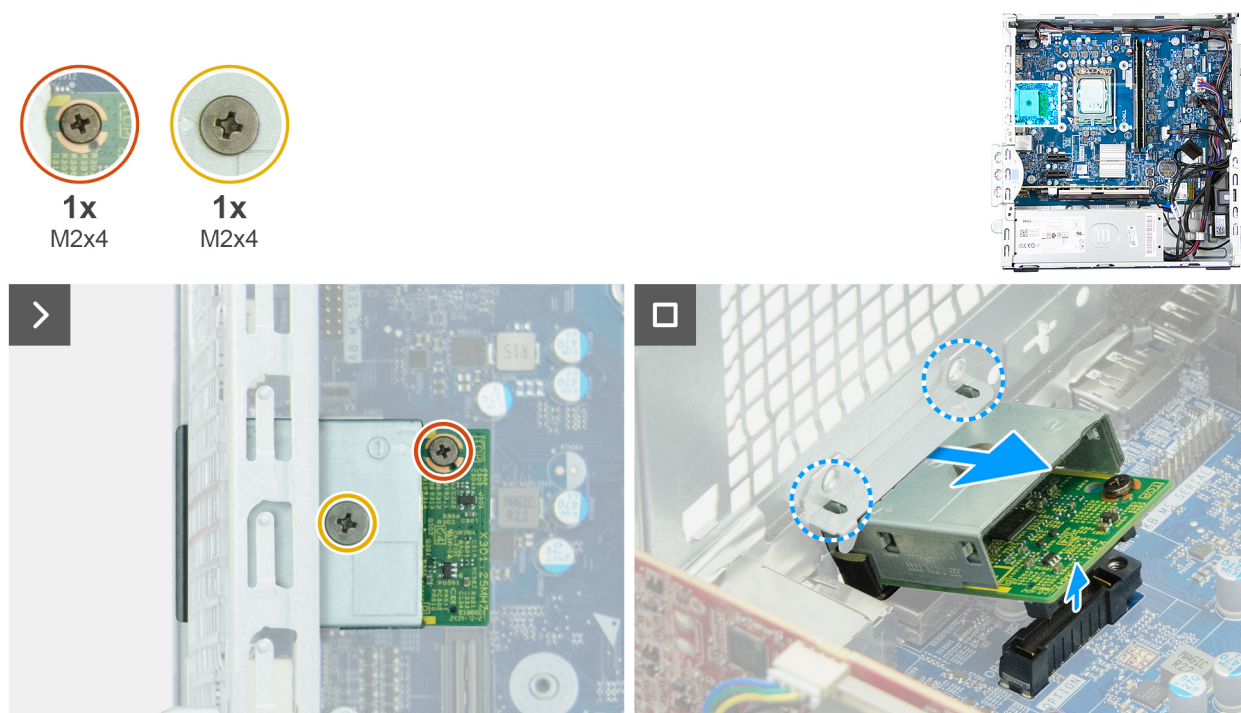
Ilustración 53. Cómo extraer el módulo de puerto opcional
