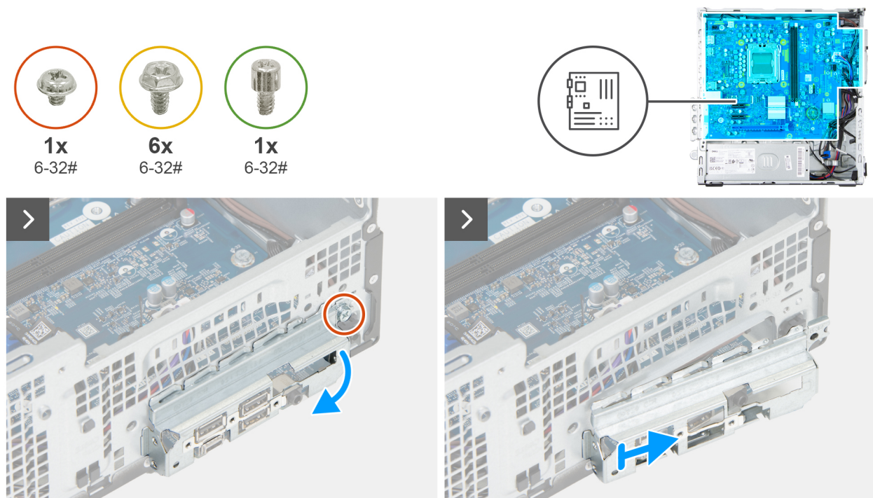
Ilustración 62. Extracción de la tarjeta madre
