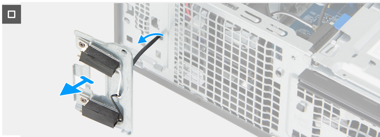
Ilustración 45. Extracción de los módulos de la antena
