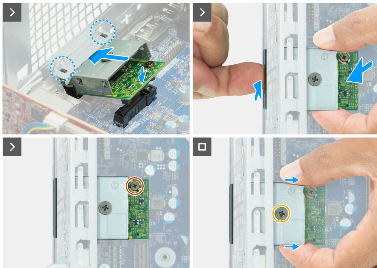
Ilustración 55. Cómo instalar el módulo de puerto opcional
