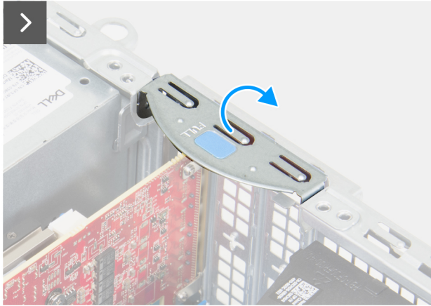
Ilustración 27. Extracción de la tarjeta gráfica
