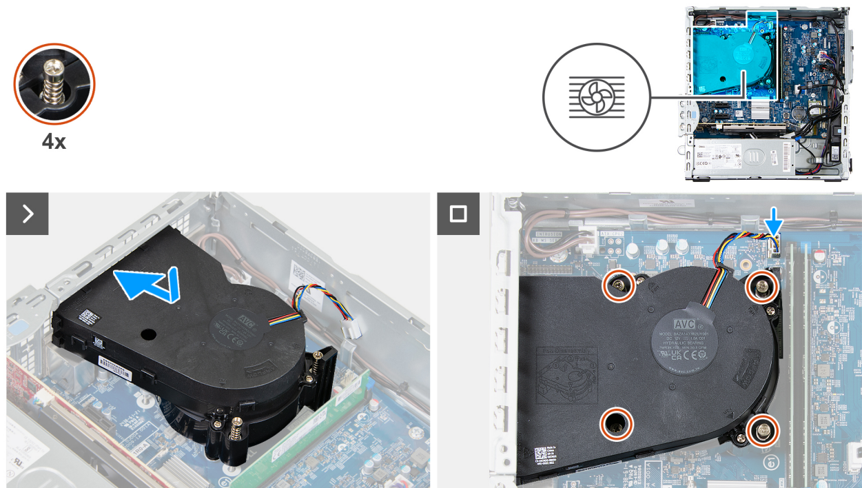
Ilustración 52. Instalación del ensamblaje del disipador de calor y el ventilador del procesador
