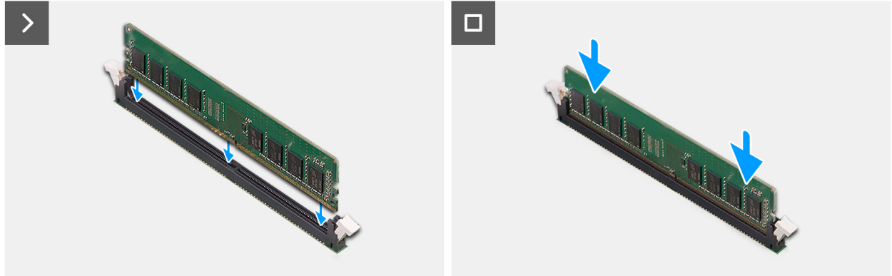
Ilustración 21. Instalación del módulo de memoria
