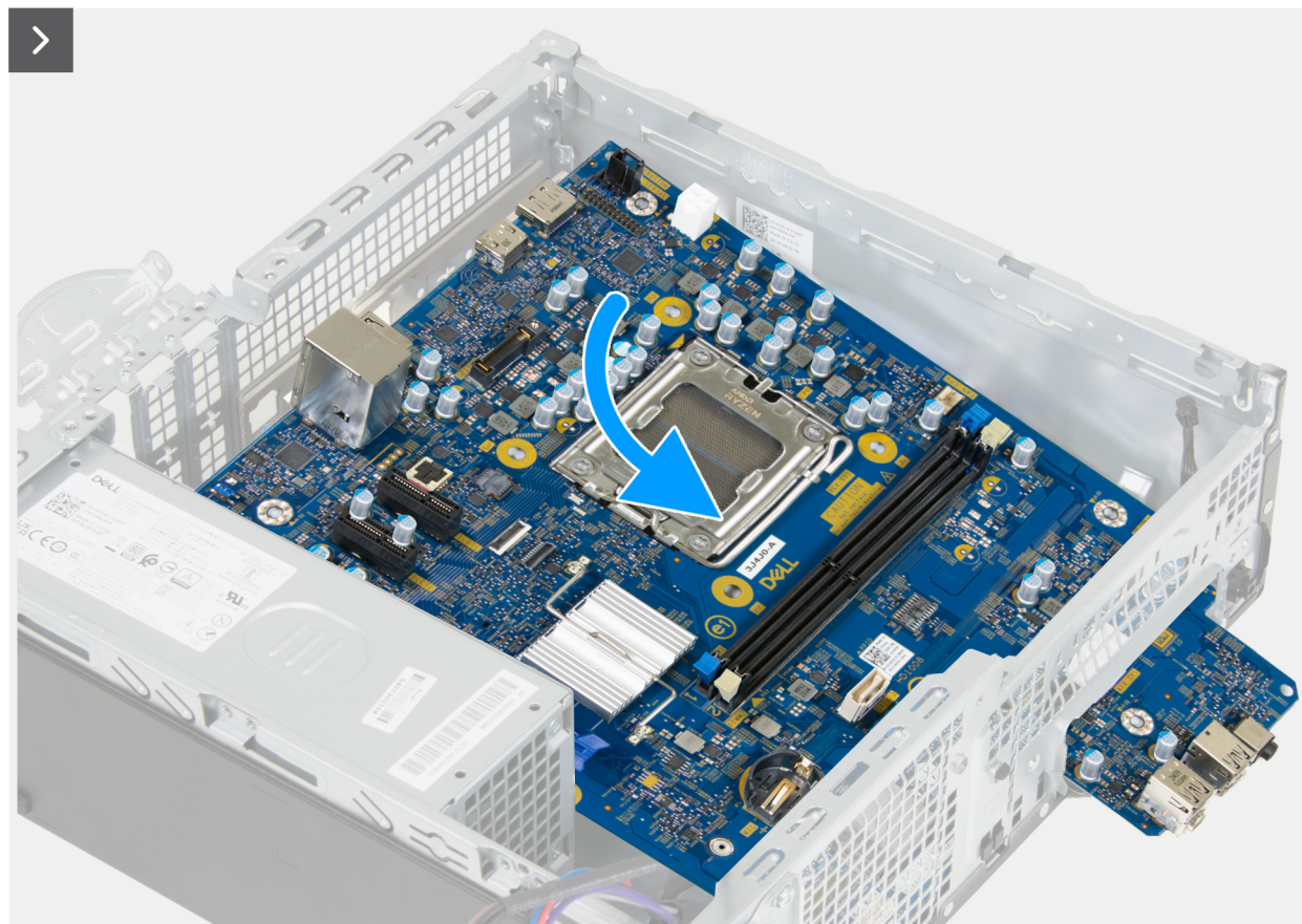
Ilustración 67. Instalación de la tarjeta madre
