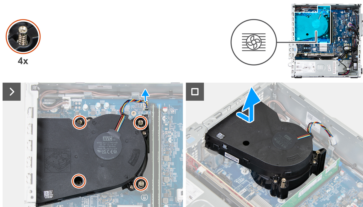
Ilustración 51. Extracción del ensamblaje del disipador de calor y el ventilador del procesador
