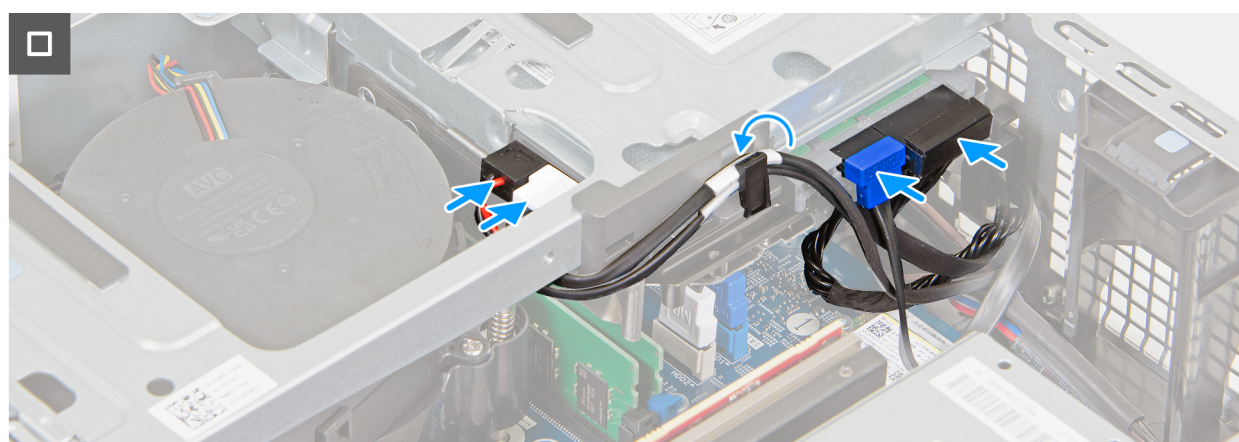
Ilustración 38. Instalación del compartimiento de la unidad
