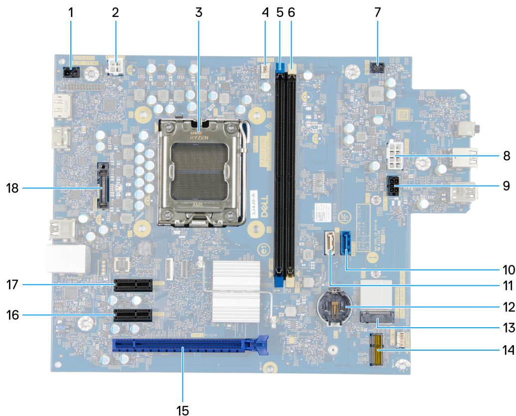
Ilustración 66. Visión general de la tarjeta madre
