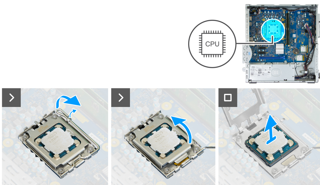
Ilustración 59. Extracción del procesador
