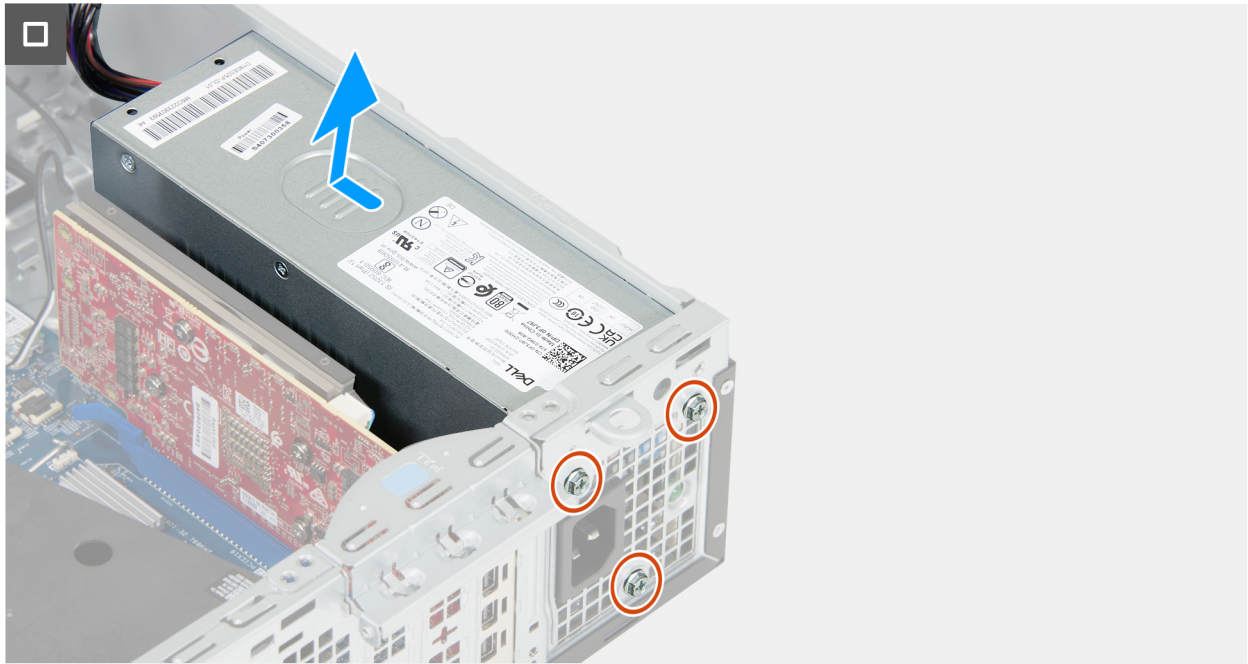
Ilustración 48. Extracción de la fuente de alimentación
