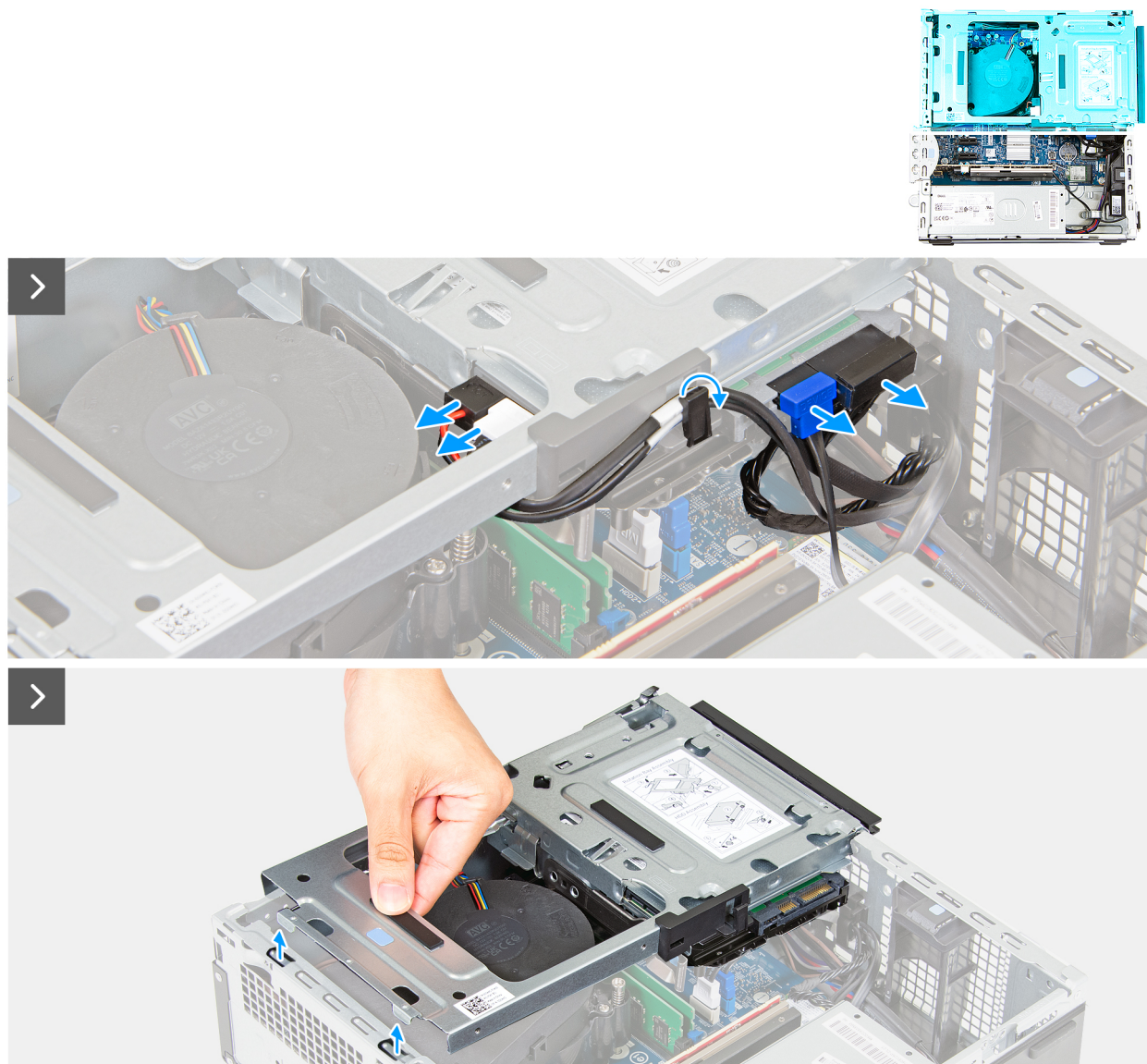
Ilustración 35. Cómo extraer el compartimiento de la unidad
