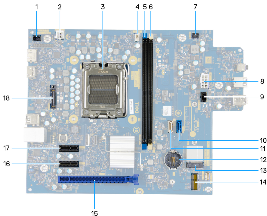
Ilustración 61. Visión general de la tarjeta madre
