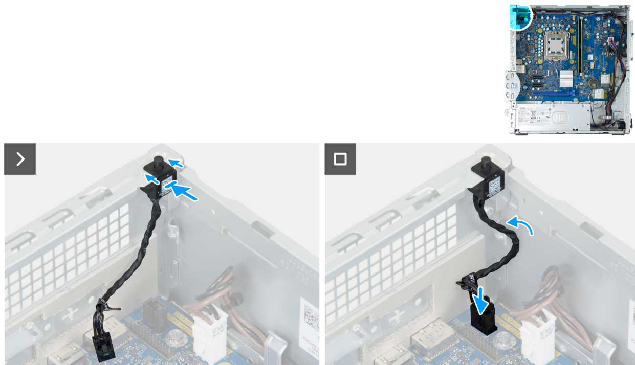
Ilustración 42. Instalación del switch de intrusión
