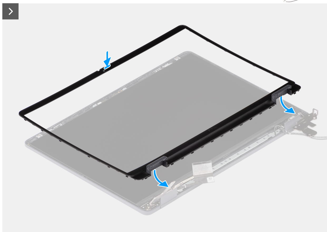
Ilustración 82. Instalación del bisel de la pantalla
