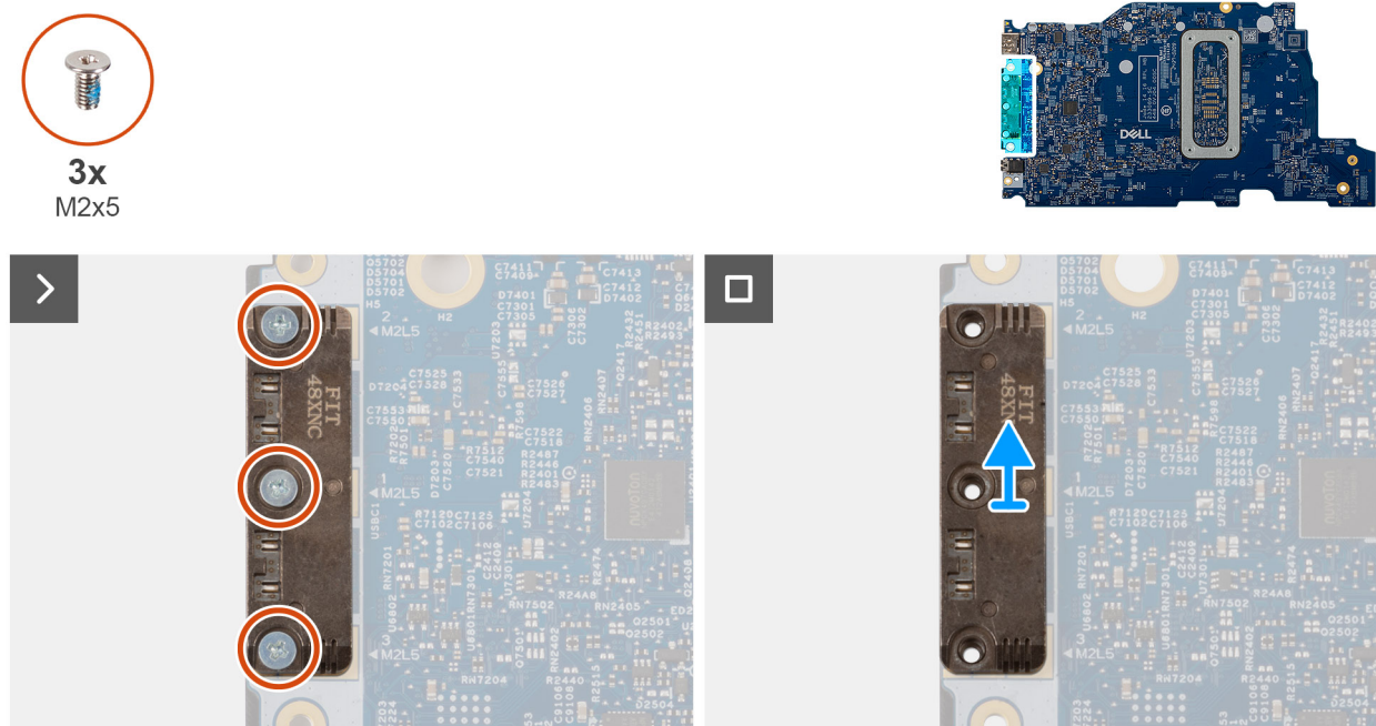
Ilustración 58. Extracción del módulo USB tipo C
