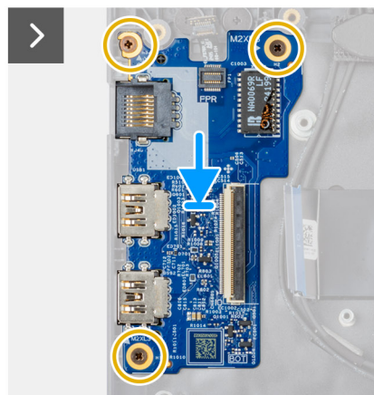
Ilustración 39. Instalación de la placa de I/O
