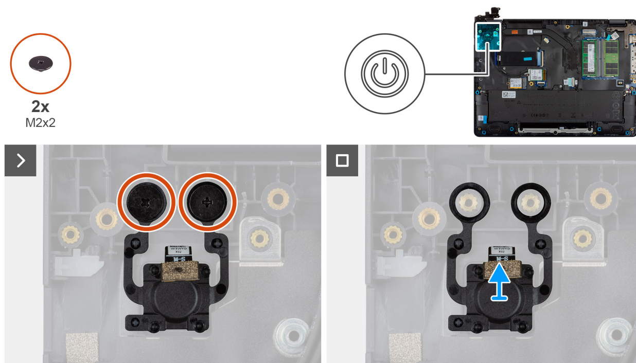
Ilustración 44. Extracción del botón de encendido con lector de huellas digitales
