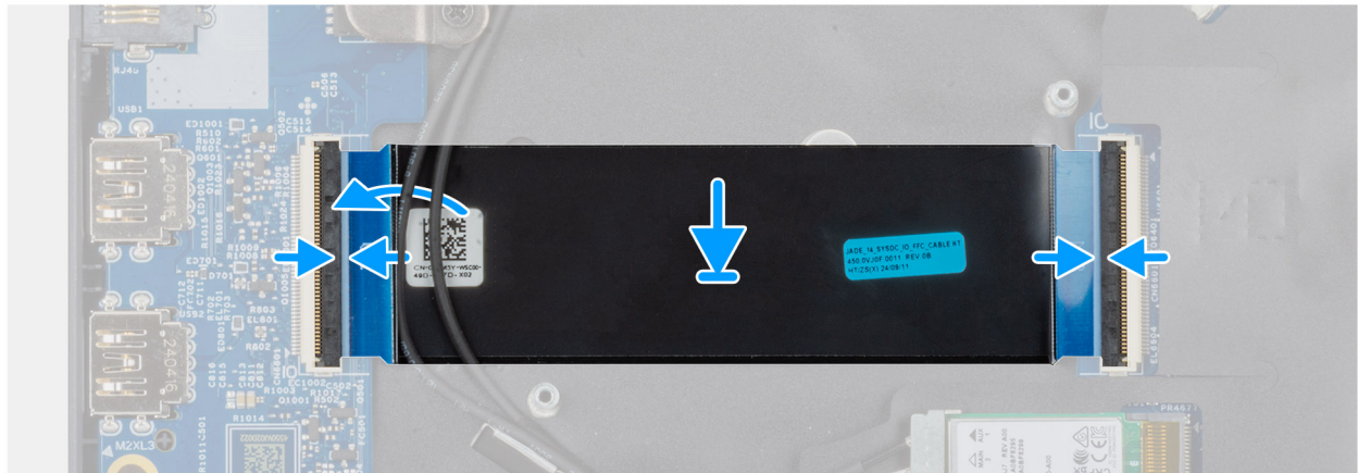
Ilustración 43. Instalación del cable FPC de la placa de I/O
