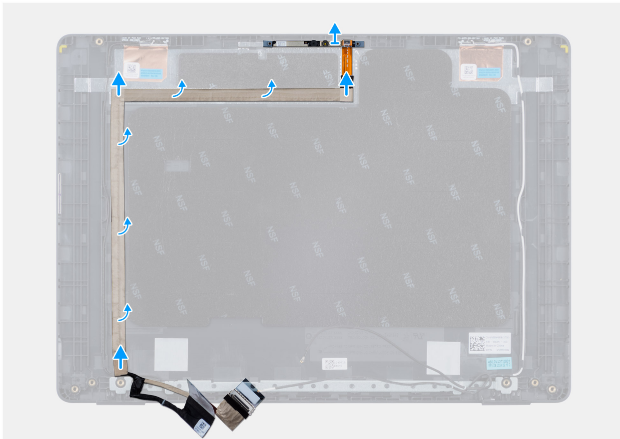
Ilustración 94. Extracción del cable de eDP
