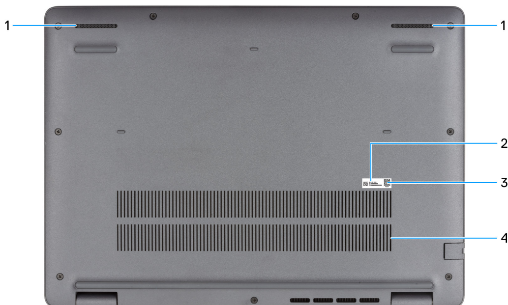
Ilustración 5. Vista inferior
