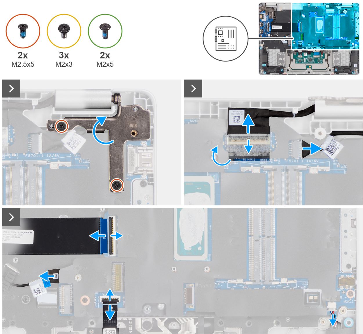
Ilustración 53. Extracción de la tarjeta madre
