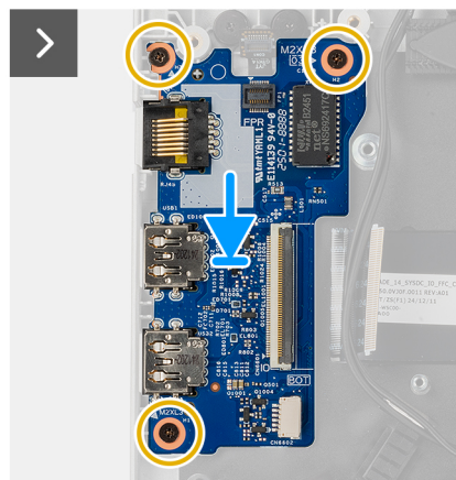
Ilustración 41. Instalación de la placa de I/O
