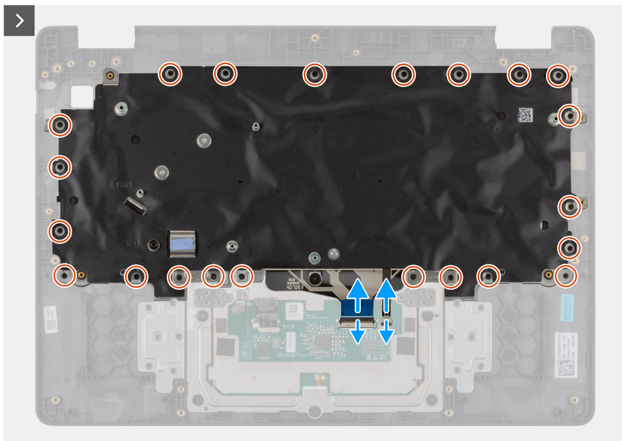
Ilustración 60. Extracción del teclado
