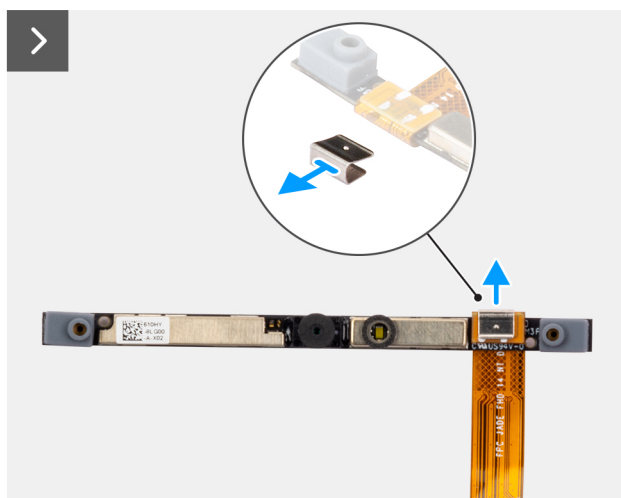
Ilustración 92. Extracción de la cámara
