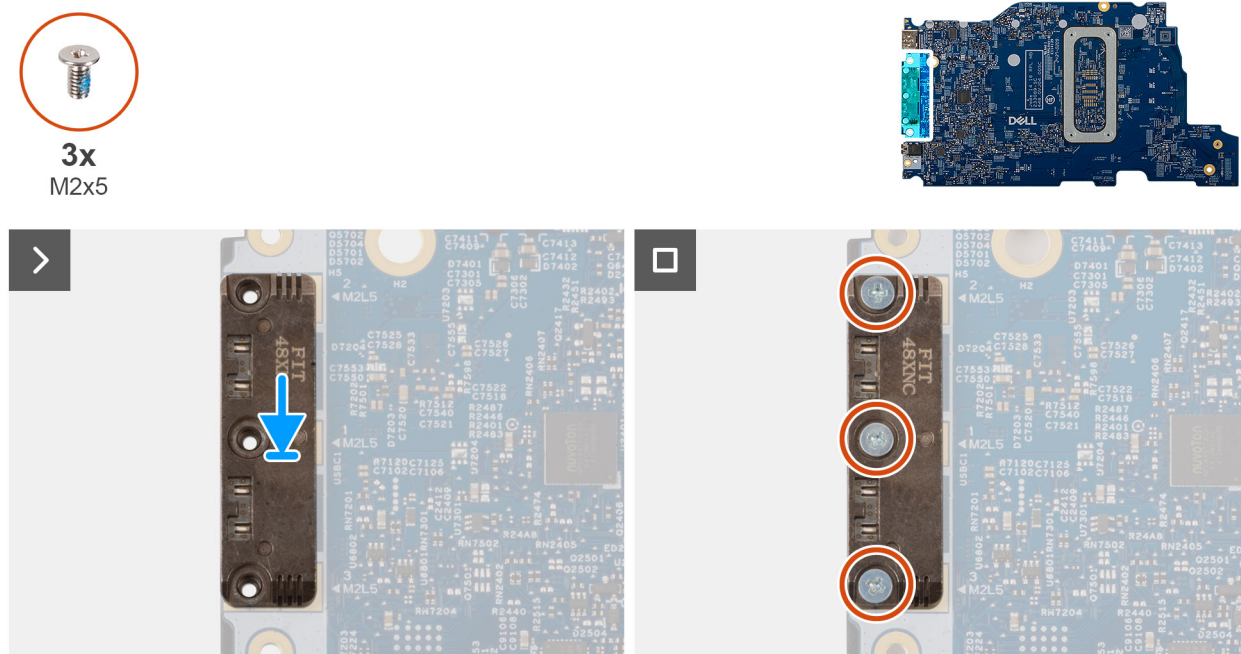
Ilustración 59. Instalación del módulo USB tipo C
