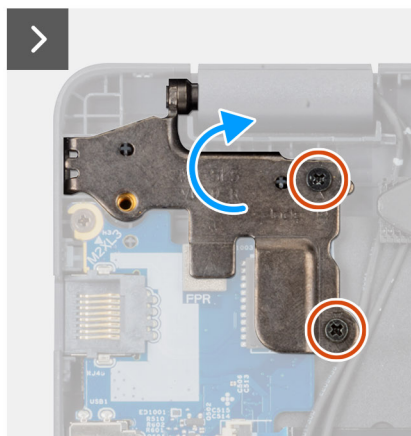
Ilustración 38. Extracción de la placa de I/O
