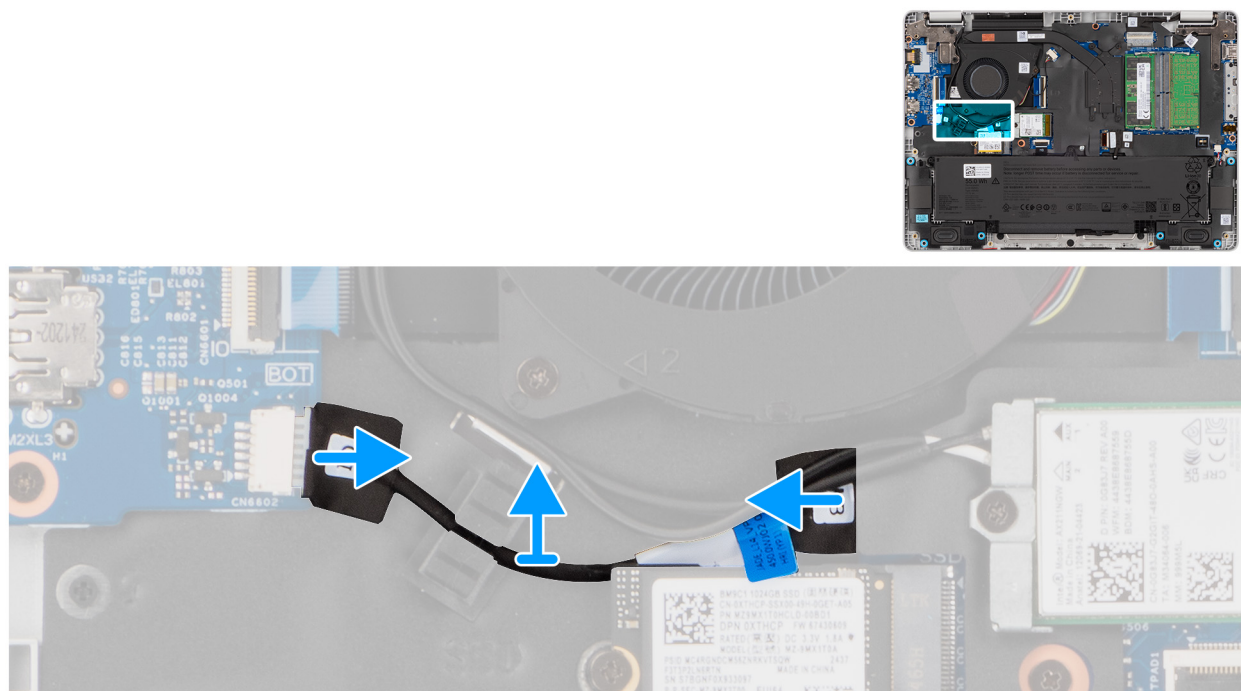
Ilustración 36. Extracción del cable vPro
