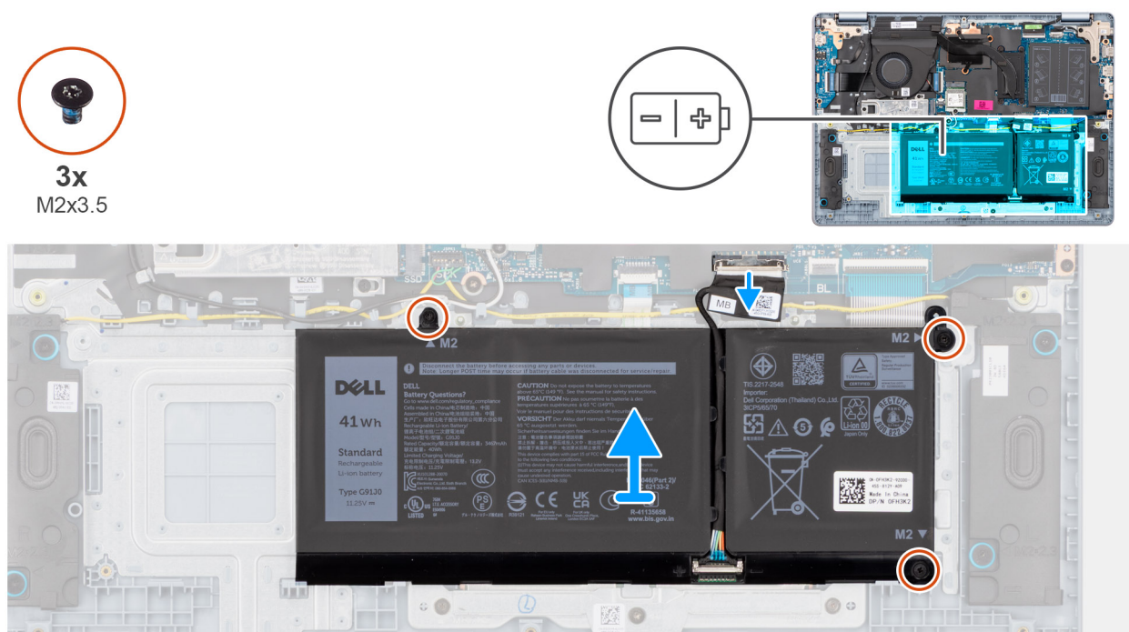
Ilustración 16. Extracción de la batería de 3 celdas
