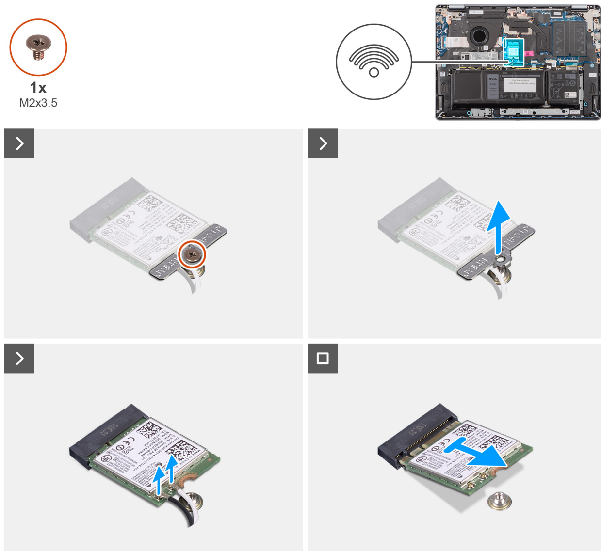
Ilustración 30. Extracción de la tarjeta inalámbrica
