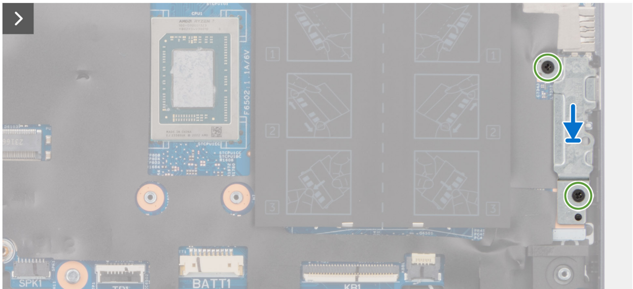
Ilustración 93. Instalación de la tarjeta madre del sistema (para computadoras enviadas con chasis de aluminio)
