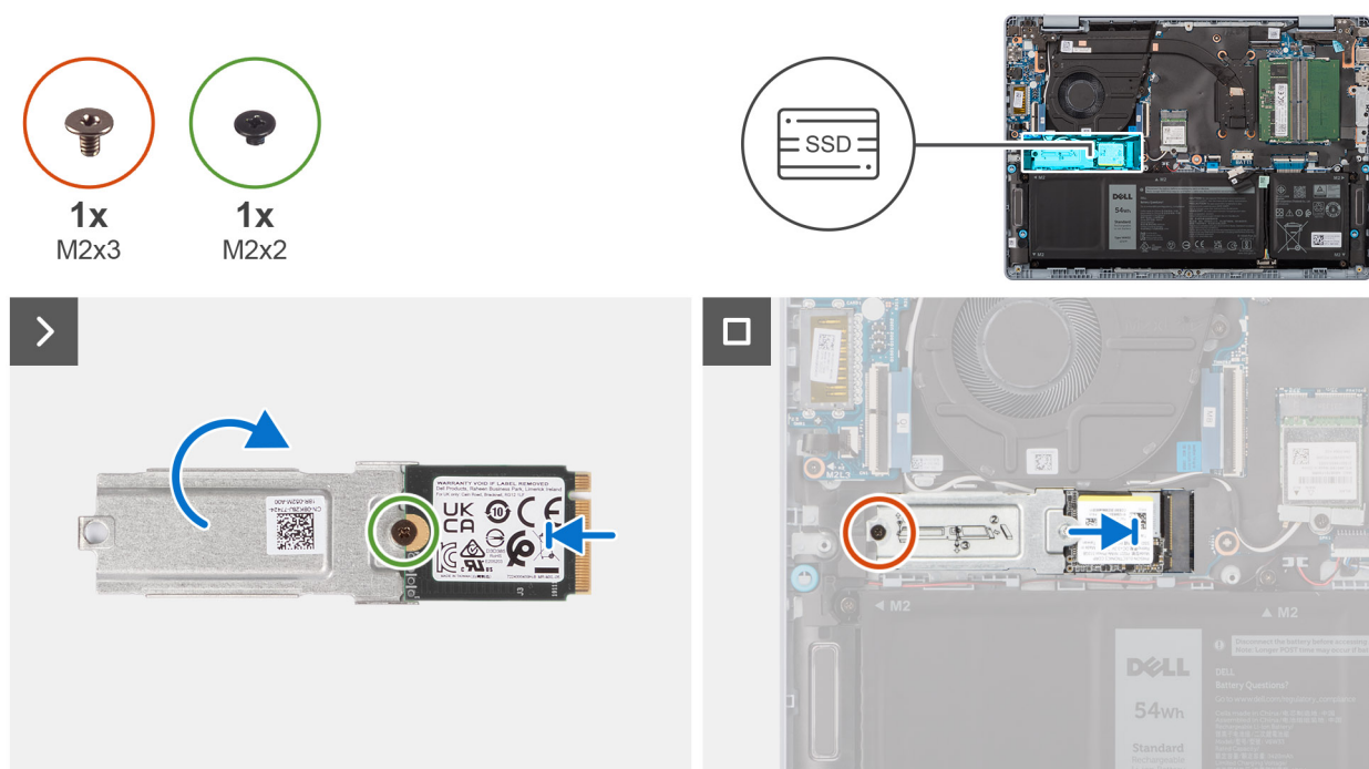
Ilustración 24. Instalación de la unidad de estado sólido
