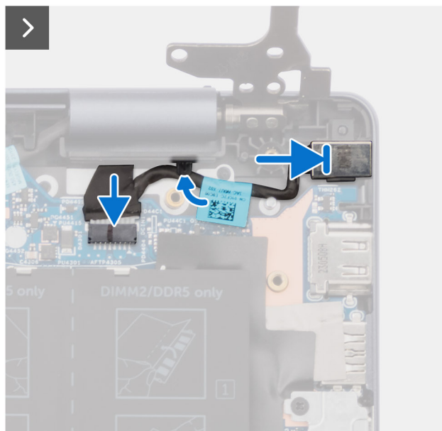
Ilustración 40. Instalación del puerto del adaptador de alimentación (para computadoras enviadas con chasis de aluminio)
