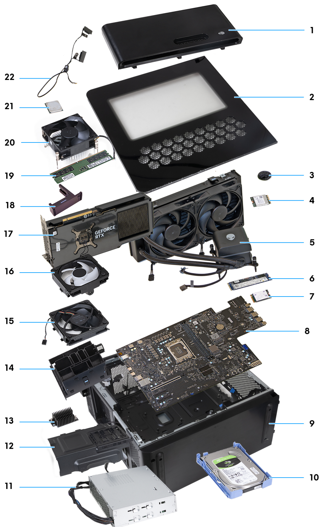
Ilustración 12. Componentes principales de Alienware Aurora ACT1250
