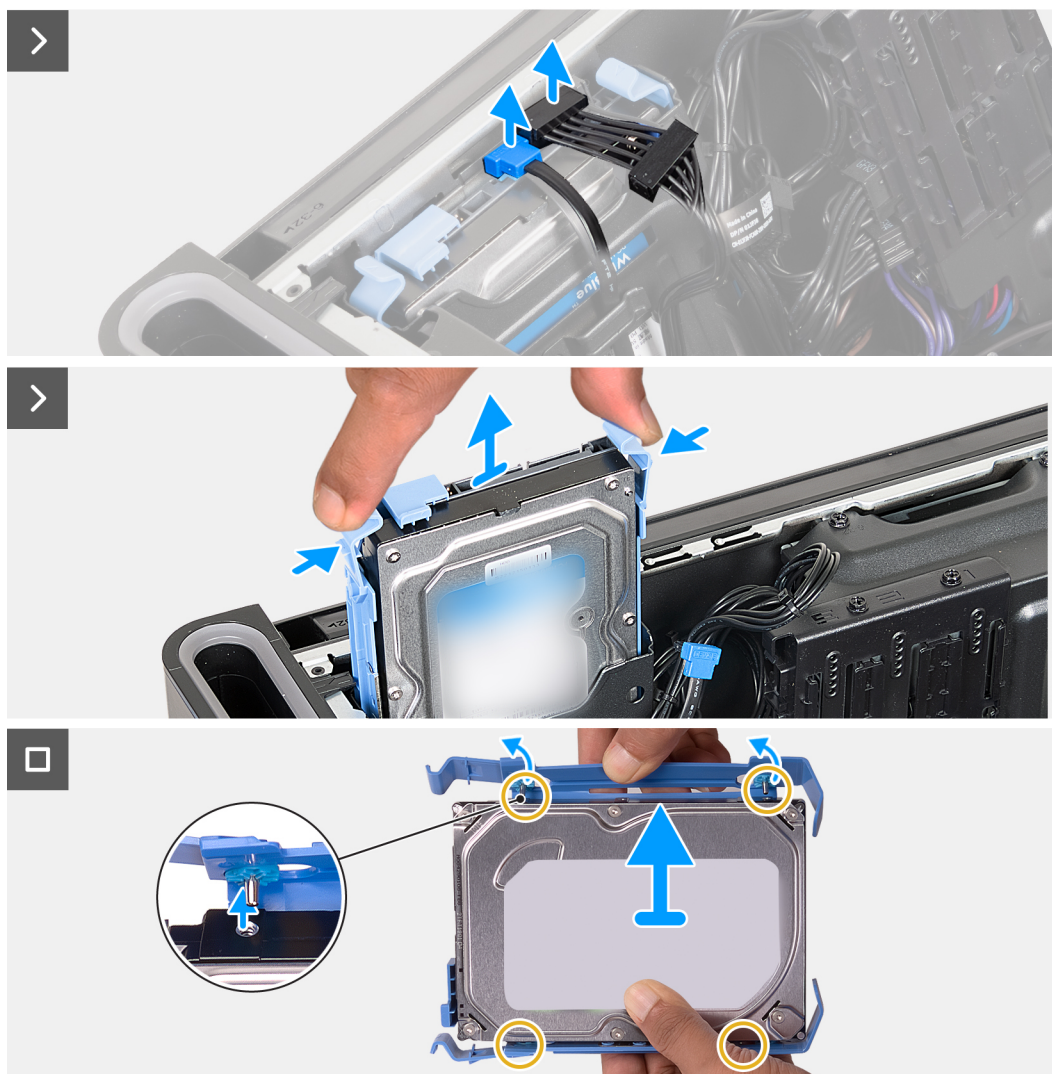
Ilustración 22. Extracción del disco duro de 3,5 pulgadas
