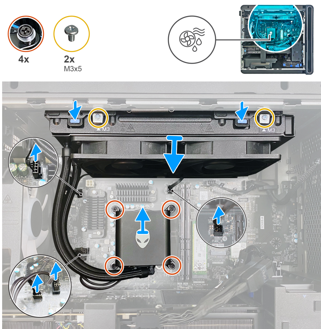
Ilustración 51. Extracción del ensamblaje de enfriamiento líquido del procesador
