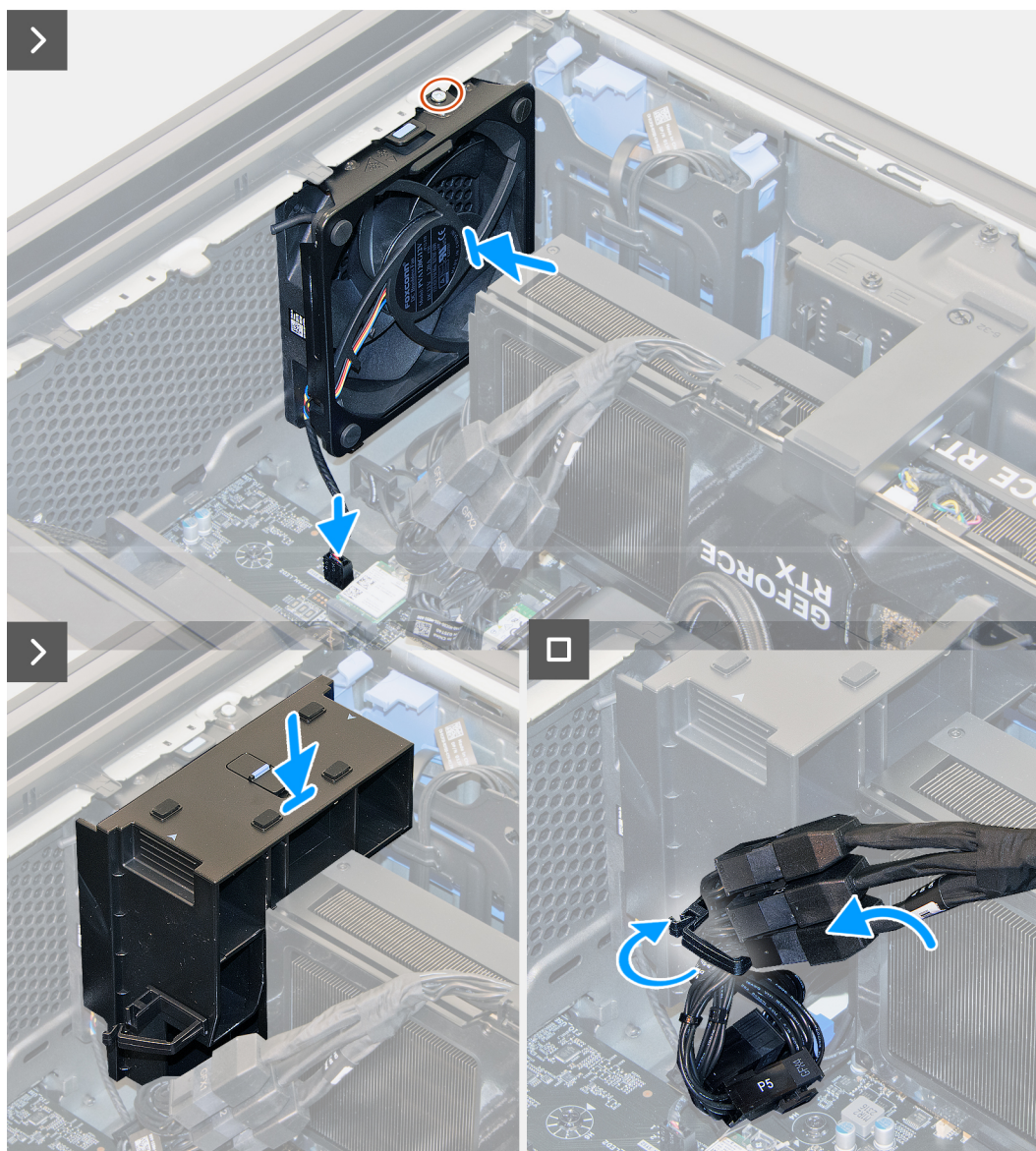
Ilustración 42. Instalación del ventilador del chasis frontal inferior
