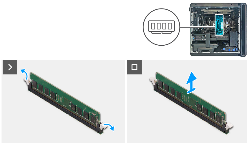
Ilustración 28. Extracción del módulo de memoria
