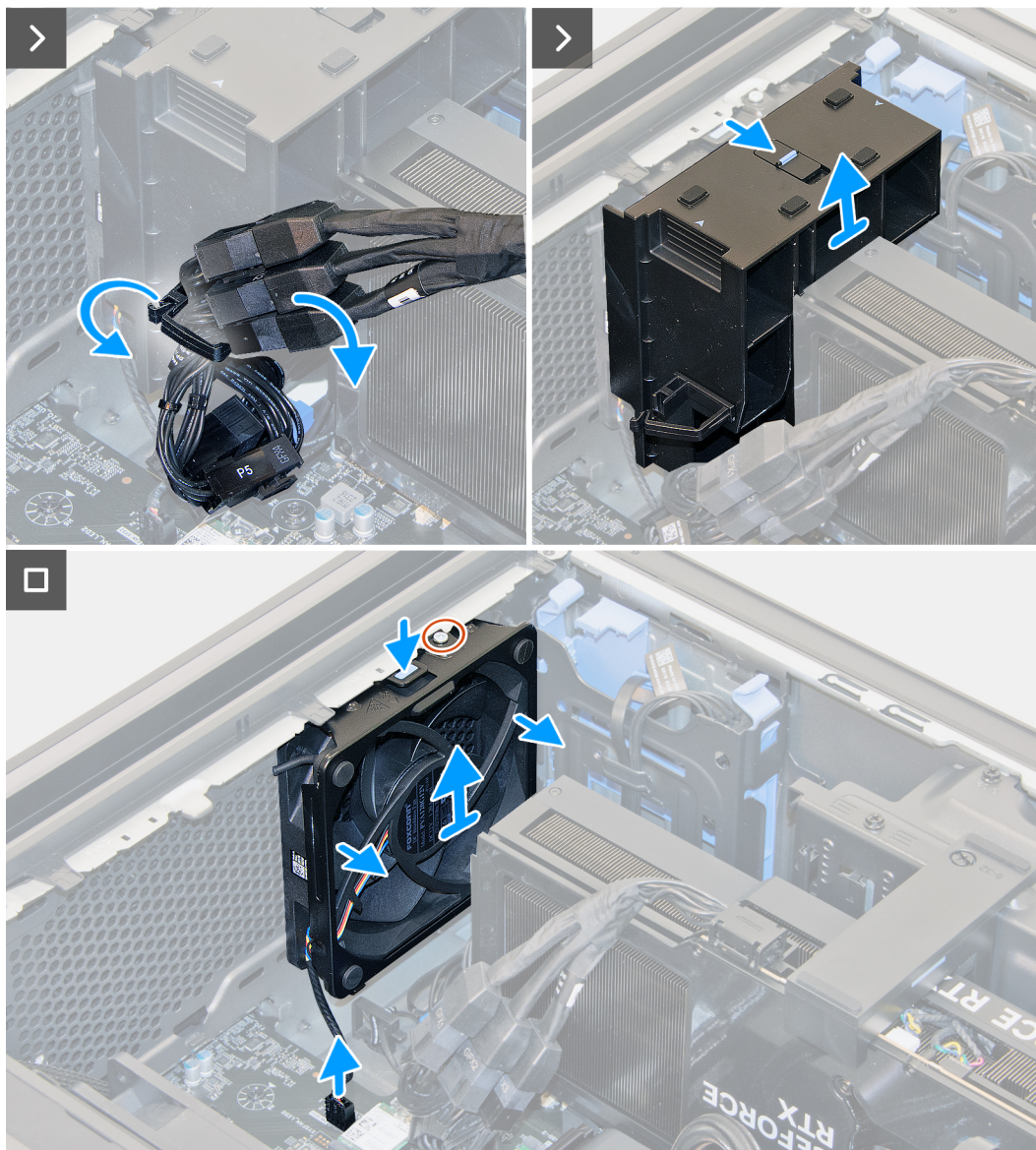
Ilustración 41. Extracción del ventilador del chasis frontal inferior
