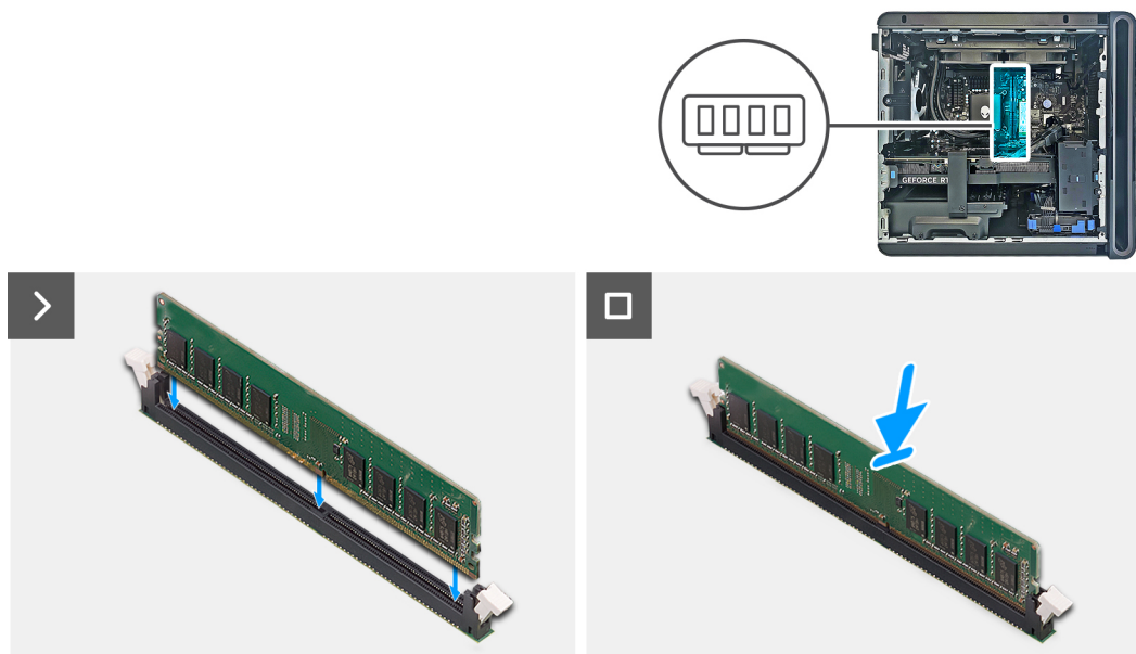
Ilustración 29. Instalación del módulo de memoria
