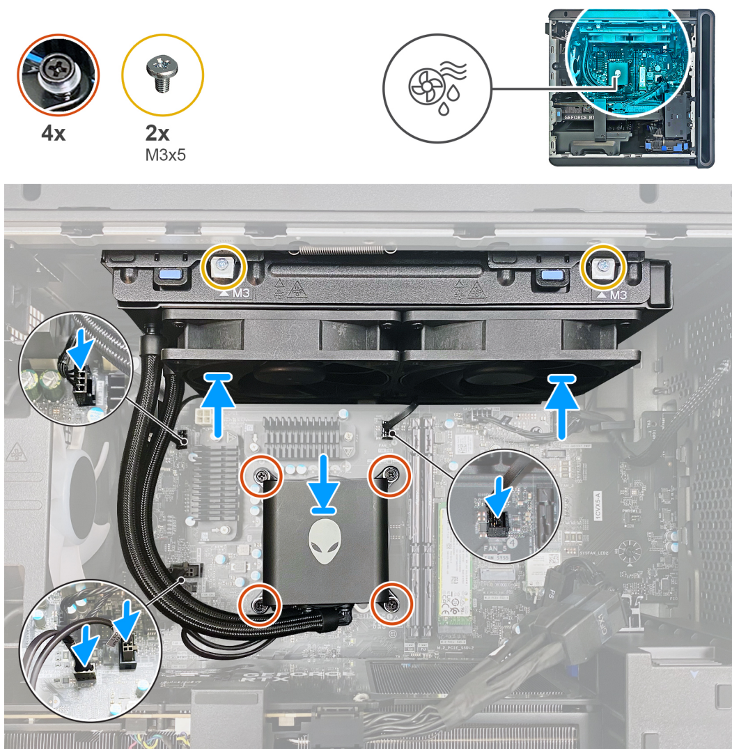
Ilustración 52. Instalación del ensamblaje de enfriamiento líquido del procesador
