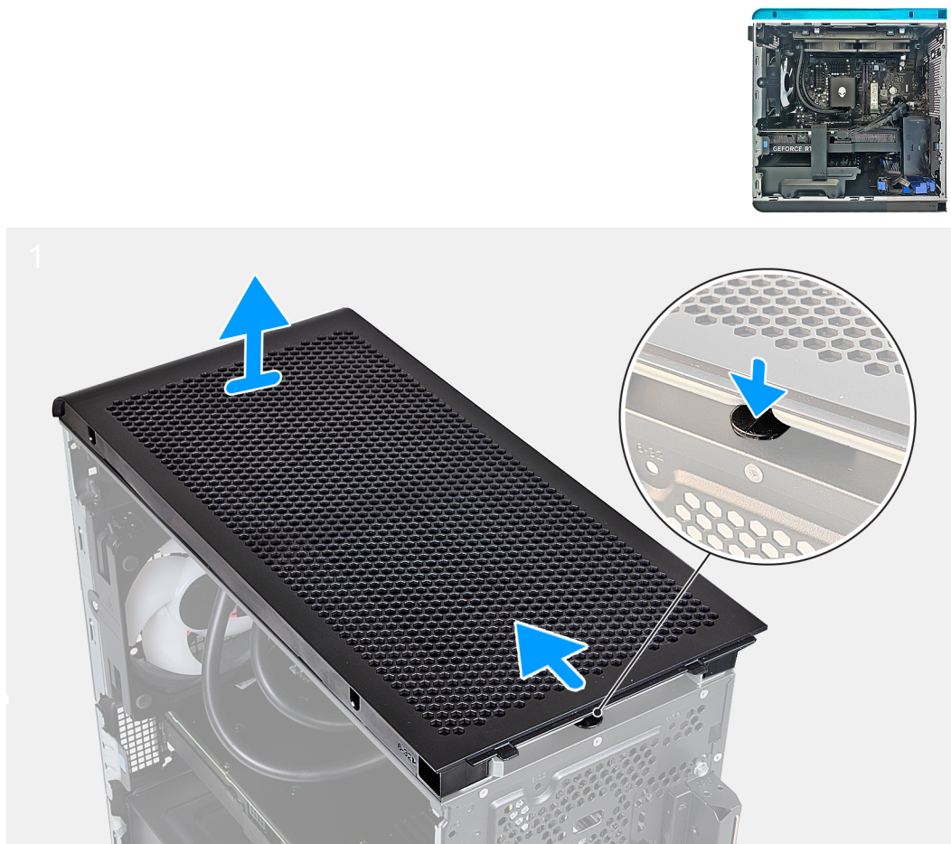
Ilustración 20. Extracción de la cubierta superior
