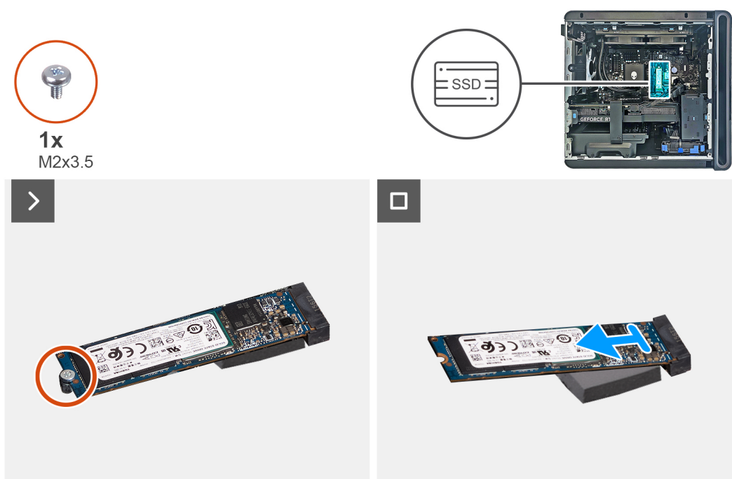
Ilustración 36. Extracción de la unidad de estado sólido M.2 2280
