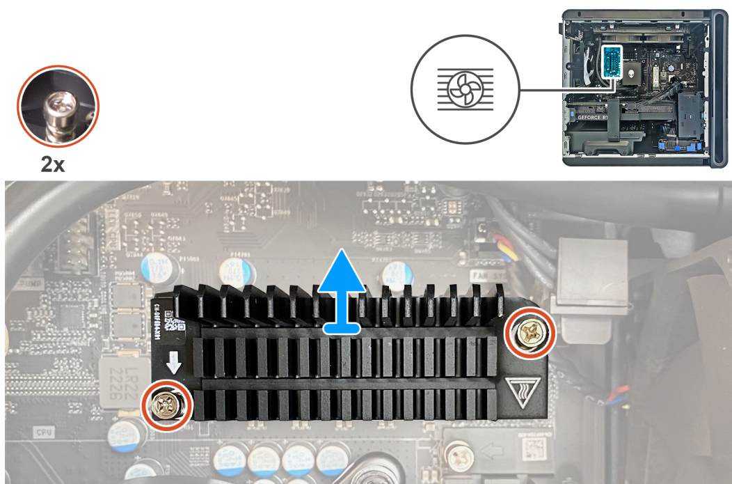
Ilustración 59. Extracción del disipador de calor de VR
