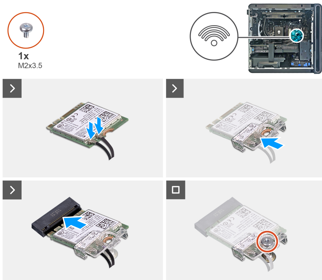
Ilustración 40. Instalación de la tarjeta inalámbrica
