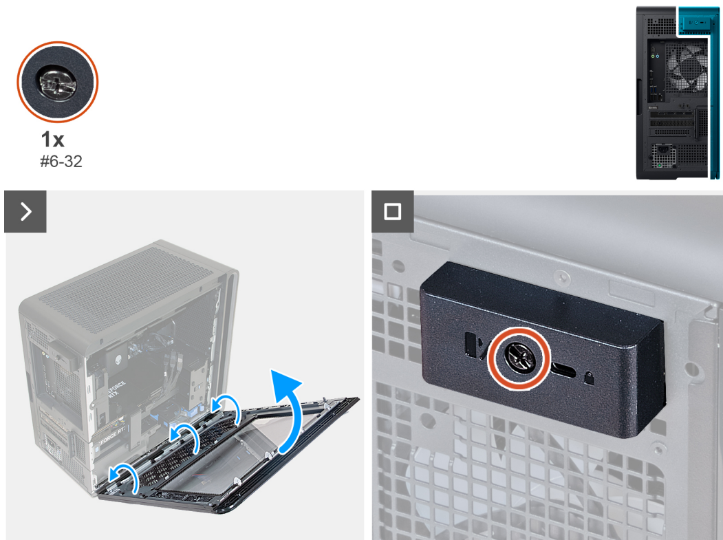
Ilustración 15. Instalación de la cubierta lateral izquierda
