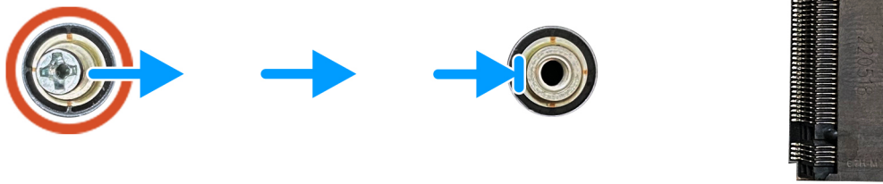
Ilustración 37. Montaje de tornillos de la unidad de estado sólido
