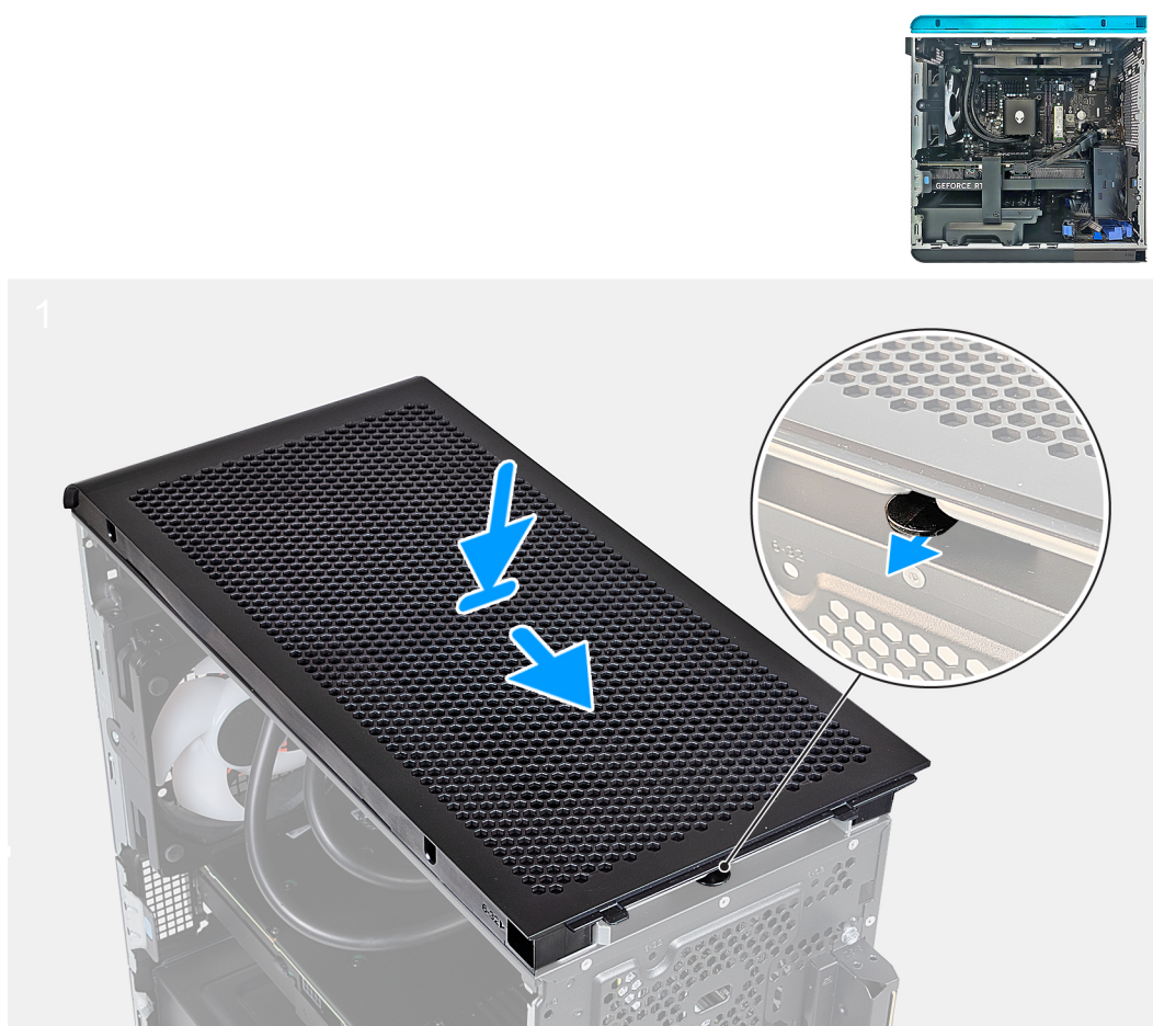
Ilustración 21. Instalación de la cubierta superior
