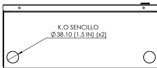
VISTA INFERIOR
