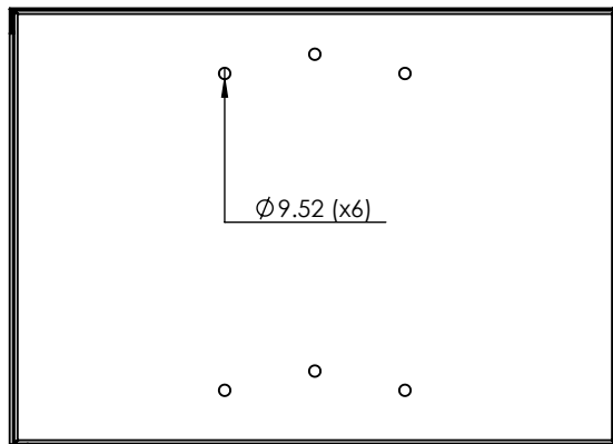
VISTA POSTERIOR
