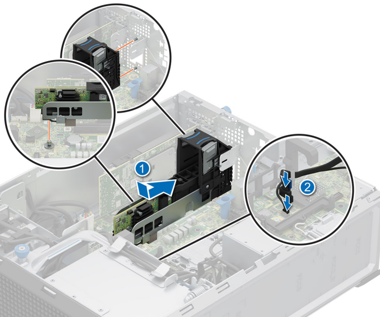
Ilustración 50. Instalación del módulo de BOSS-N1
