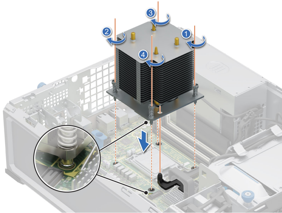
Ilustración 41. Instalación del disipador de calor
