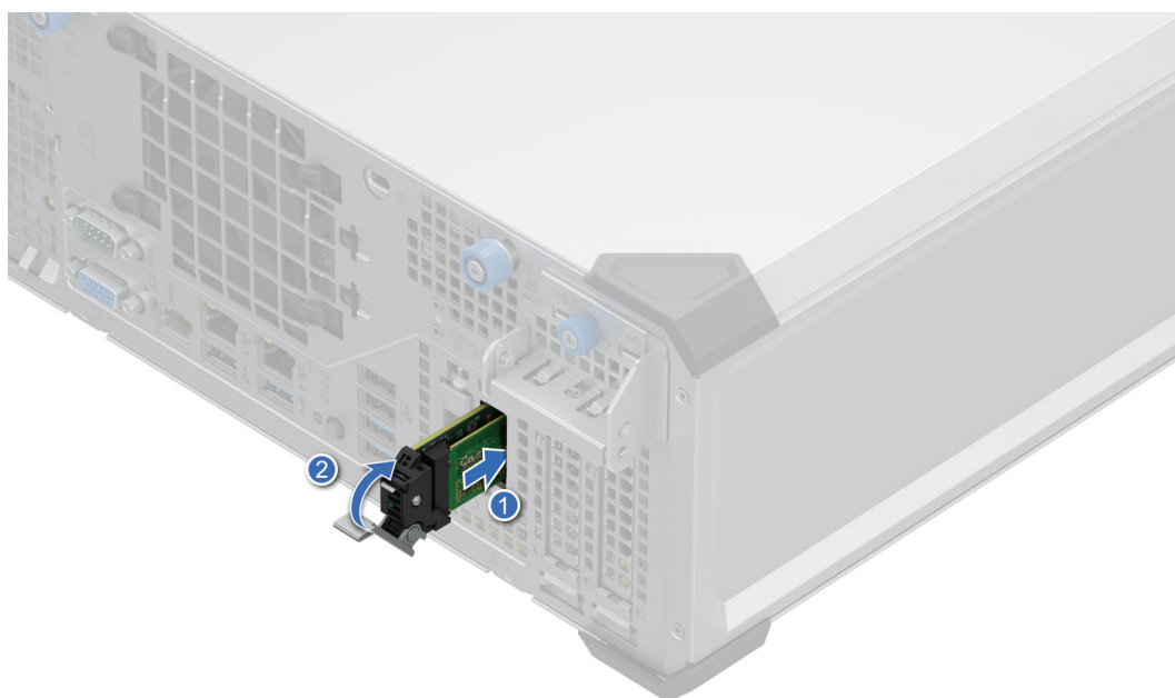
Ilustración 56. Instalación del portatarjetas de BOSS-N1
