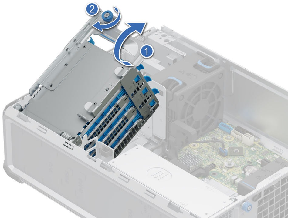
Ilustración 22. Instalación de un portaunidades
