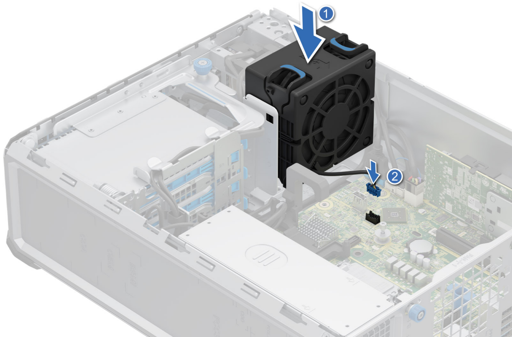
Ilustración 29. Instalación del ventilador de PCI de alto rendimiento (HPR)
