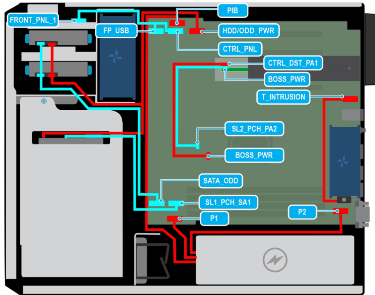
Ilustración 32. Colocación de cables: 3 SATA con chip de 3,5 pulgadas + 2 SATA con chip de 2,5 pulgadas
