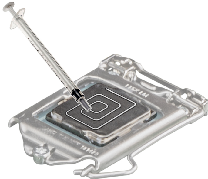
Ilustración 40. Aplicación de la pasta térmica en la parte superior del procesador
