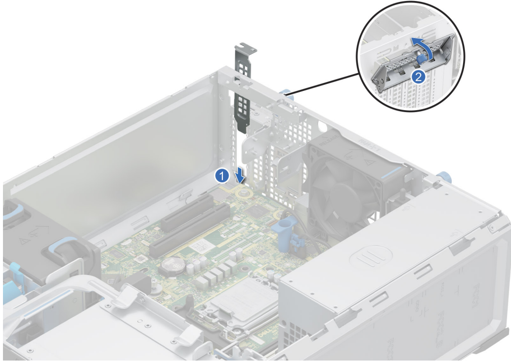
Ilustración 44. Instalación del soporte de relleno metálico
