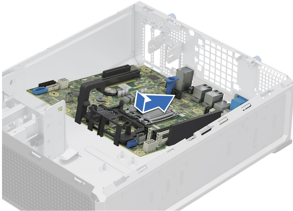
Ilustración 63. Instalación de la tarjeta madre
