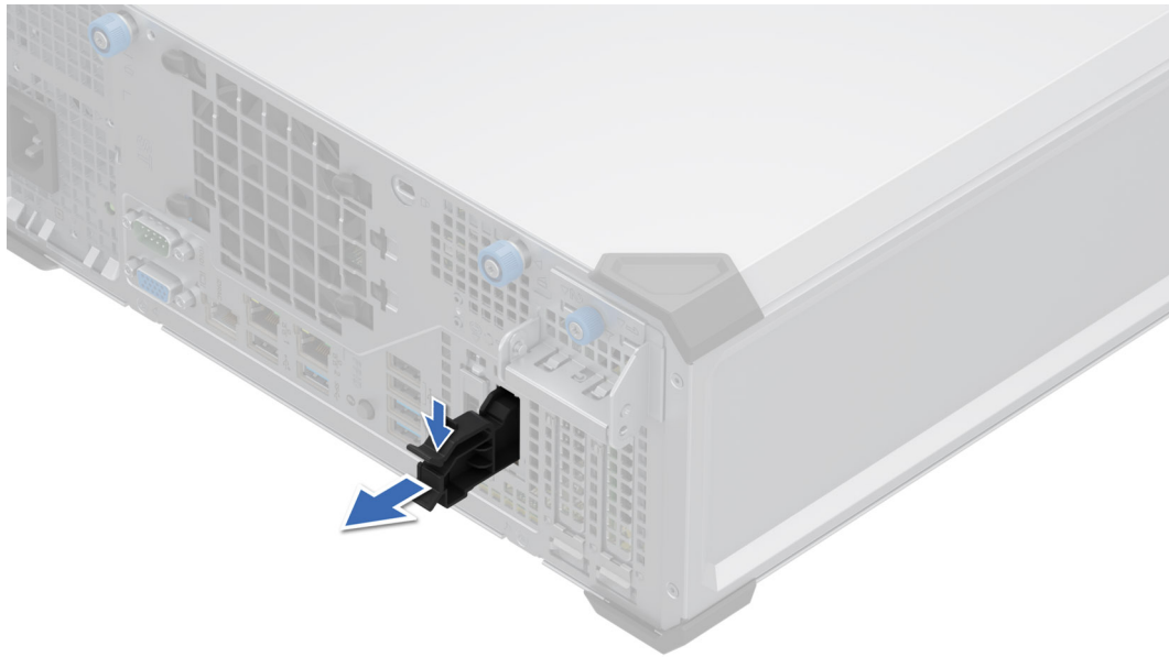
Ilustración 49. Extracción del módulo de BOSS-N1 de relleno
