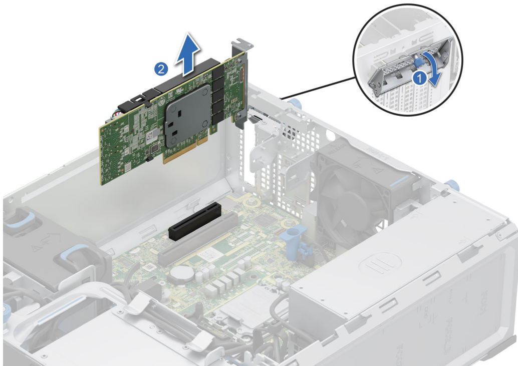
Ilustración 43. Extracción de una tarjeta de expansión
