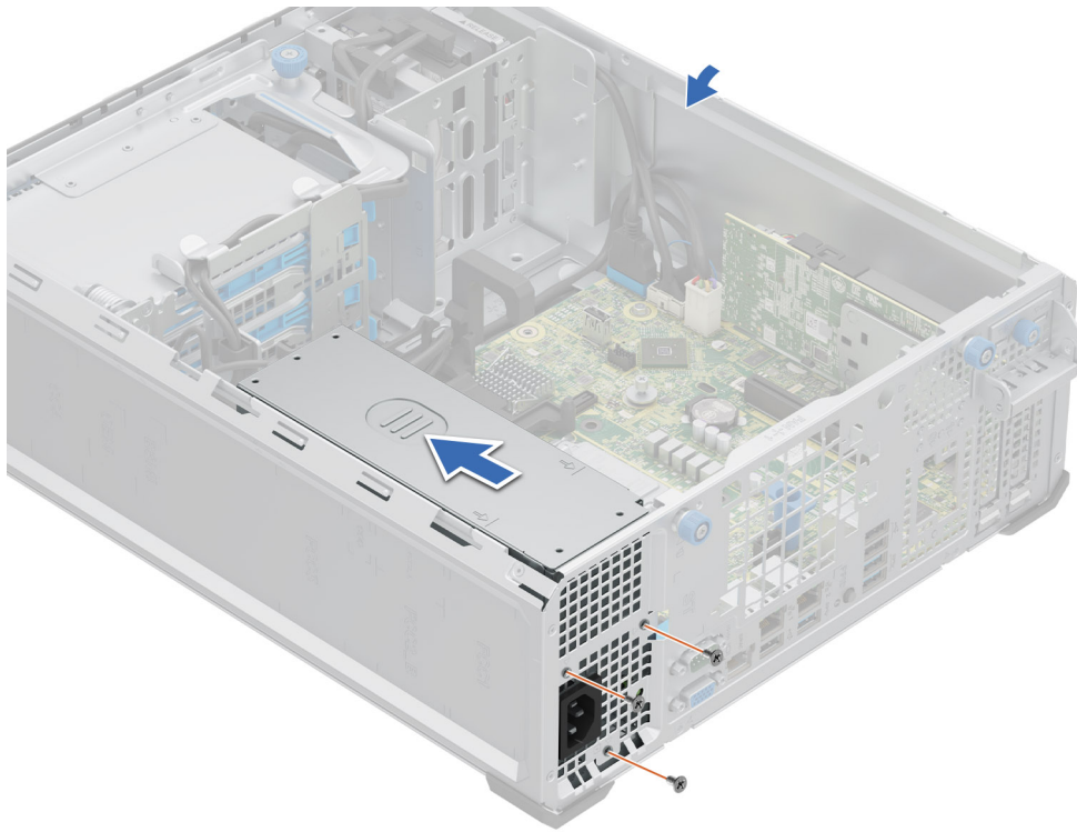
Ilustración 57. Extracción de la PSU cableada
