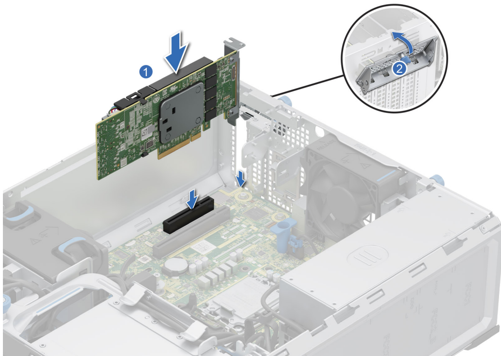
Ilustración 46. Instalación de una tarjeta de expansión
