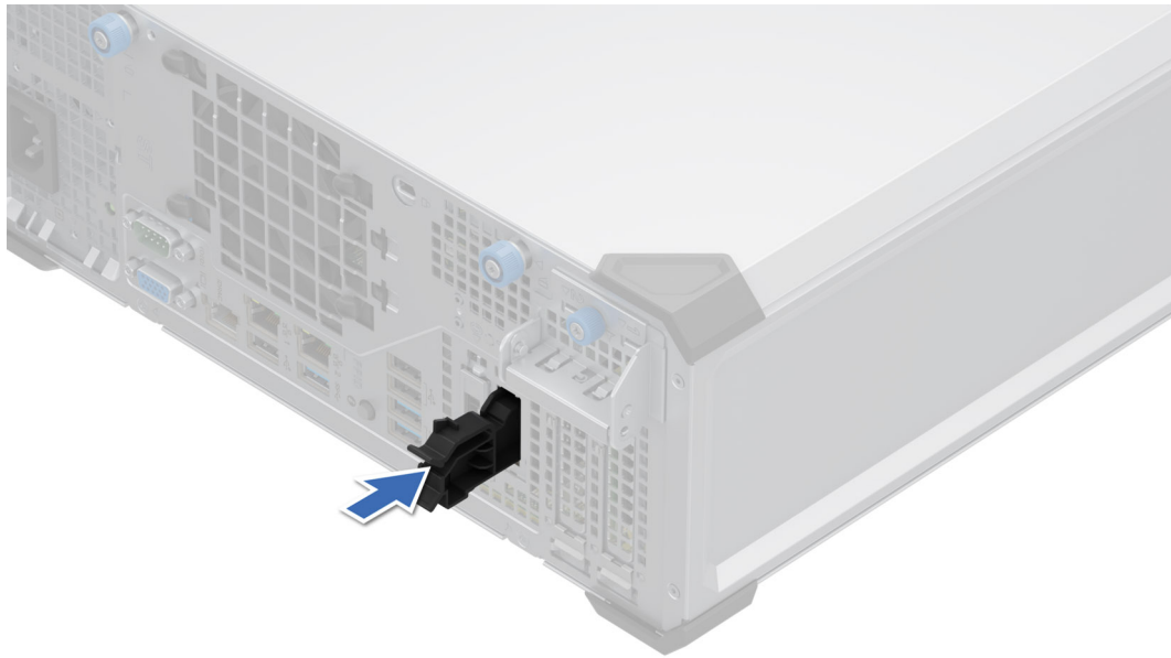
Ilustración 53. Instalación del portaunderes de tarjeta BOSS-N1 de relleno
