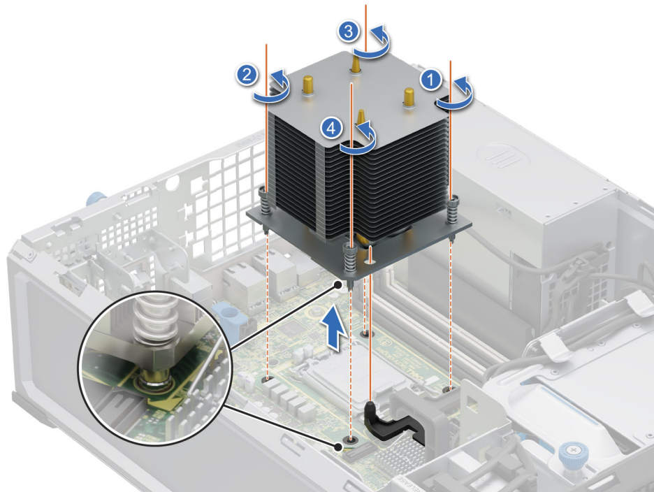
Ilustración 37. Extracción del disipador de calor
