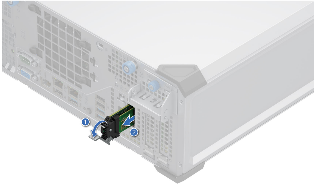
Ilustración 51. Extracción del portatajadas de tarjeta BOSS-N1
