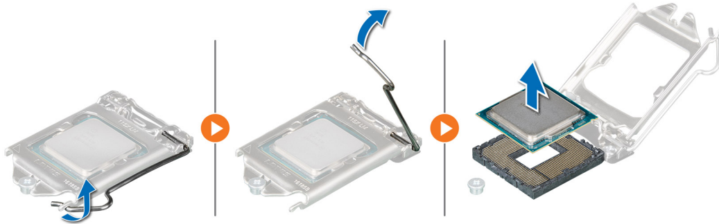
Ilustración 38. Extracción del procesador
