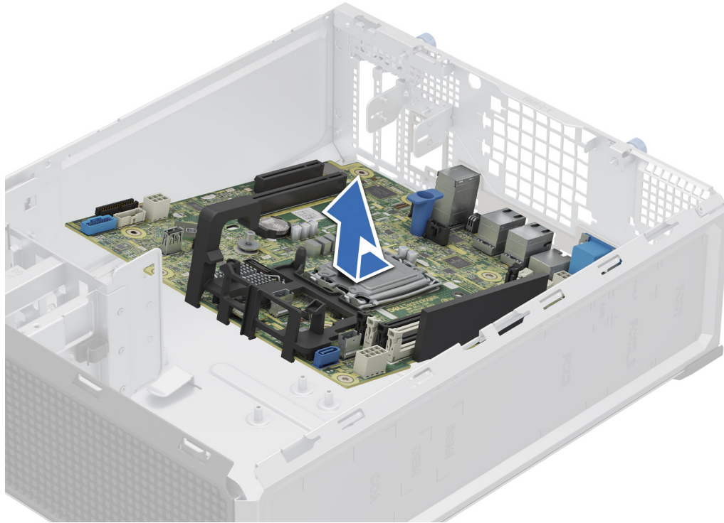
Ilustración 62. Extracción de la tarjeta madre
