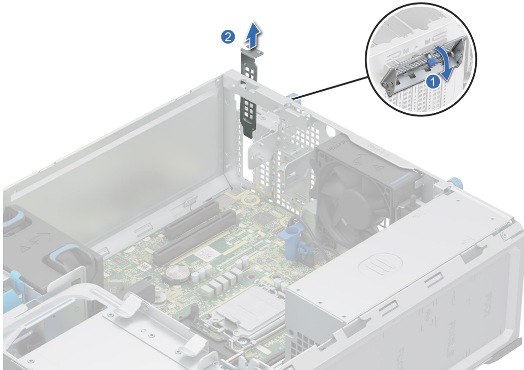
Ilustración 45. Extracción del soporte de relleno metálico
