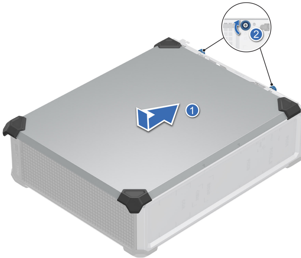
Ilustración 13. Instalación de la cubierta del sistema
