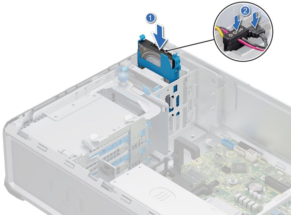
Ilustración 23. Instalación de un portaunidades
