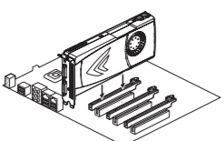
Billede 1: Tilslutning af videokortet til ekspansionsporten på moderkortet.
