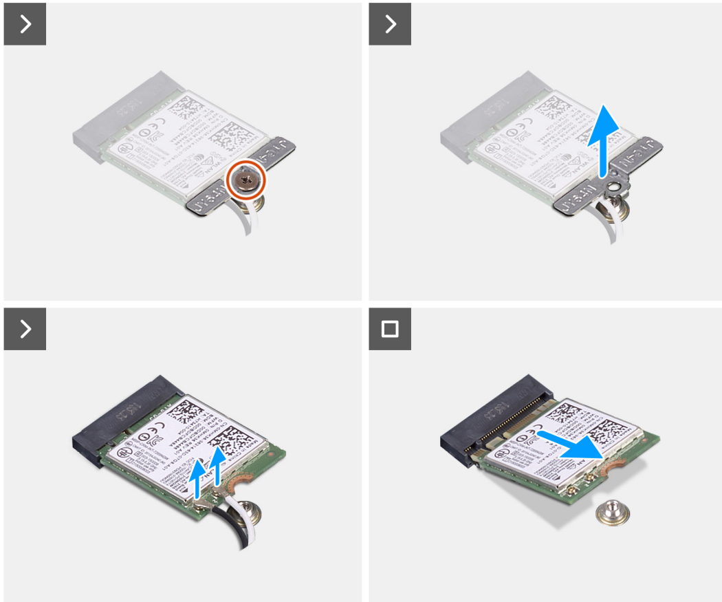
Ilustración 14. Extracción de la tarjeta inalámbrica
