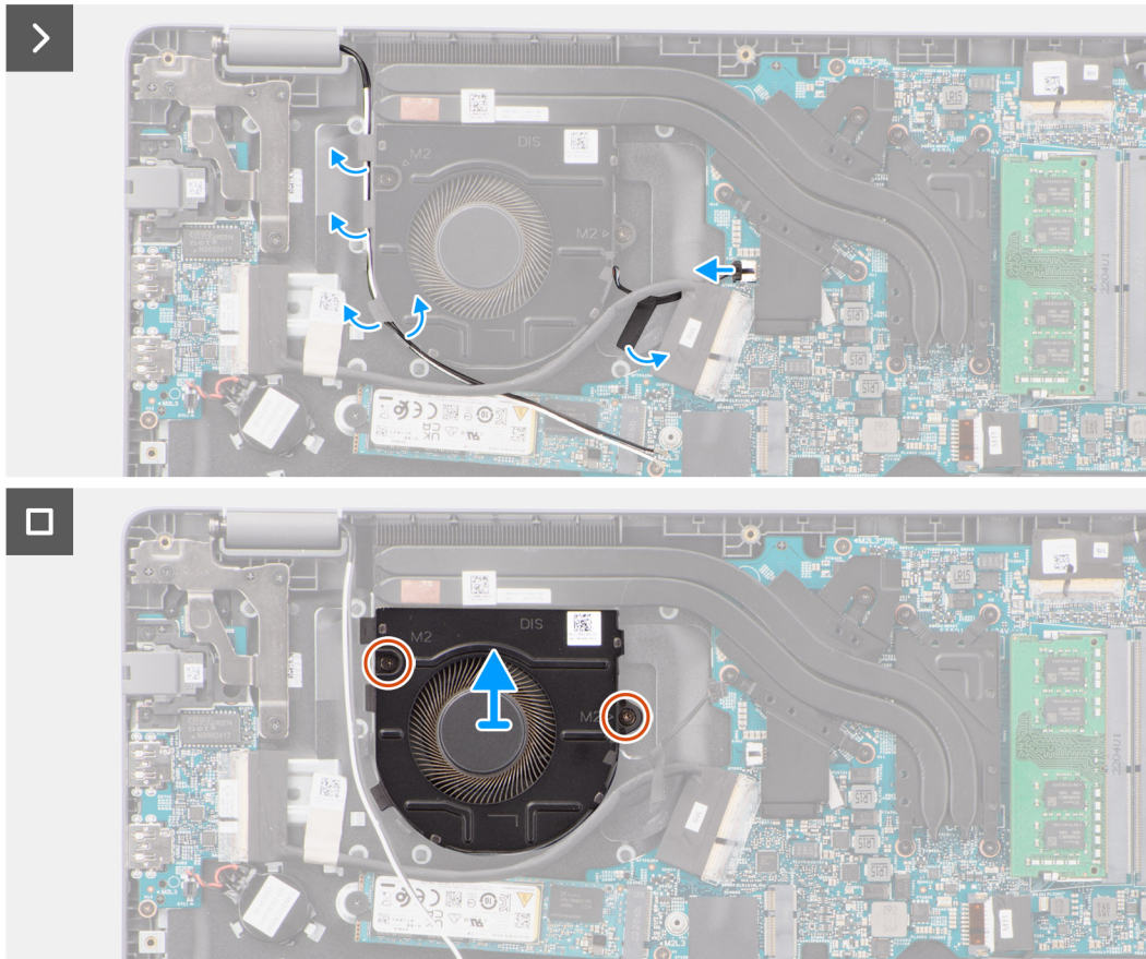
Ilustración 33. Extracción del ventilador
