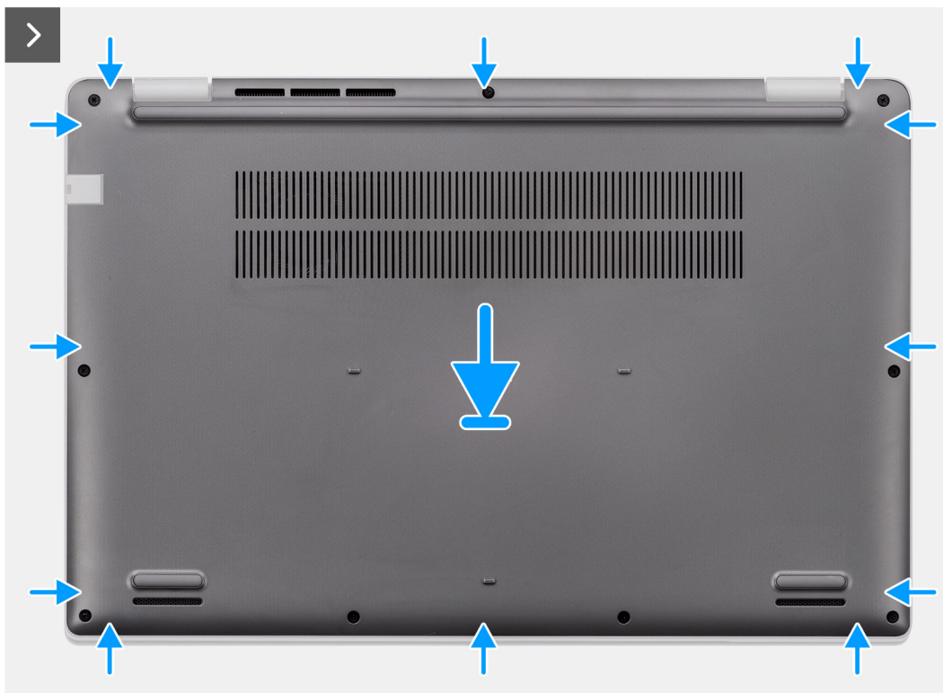
Ilustración 10. Instalación de la cubierta de la base
