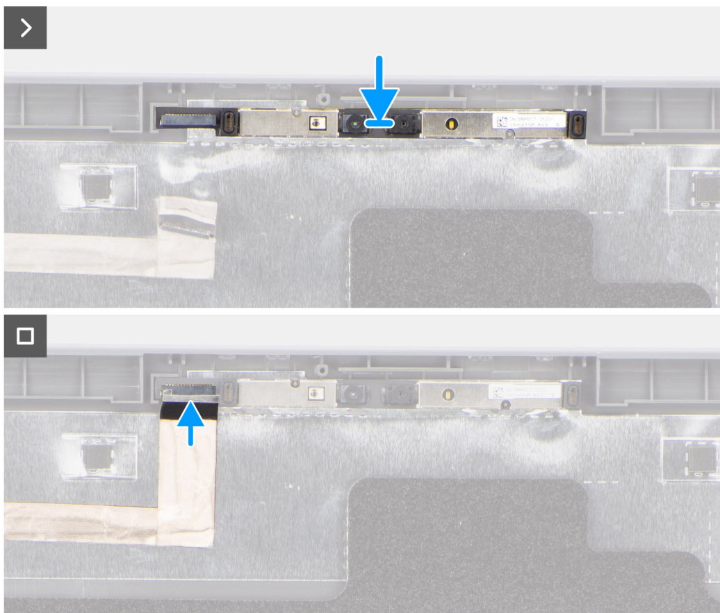
Ilustración 67. Instalación de la cámara
