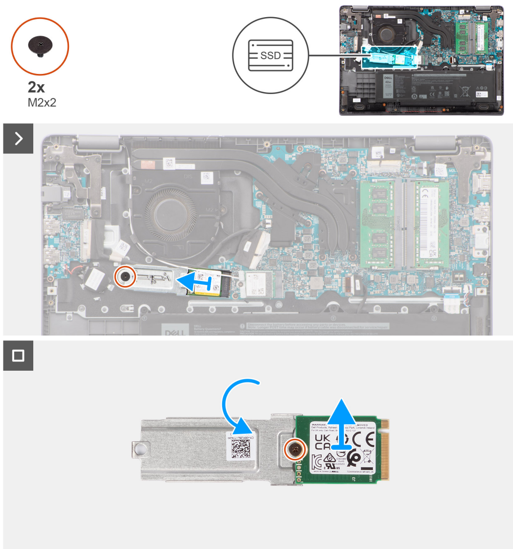
Ilustración 22. Extracción de la unidad de estado sólido M.2 2230
