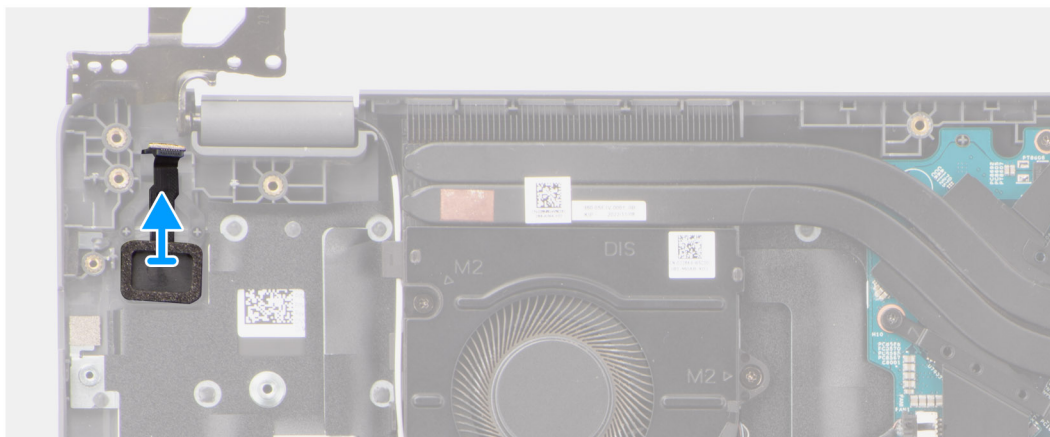
Ilustración 39. Extracción del botón de encendido
