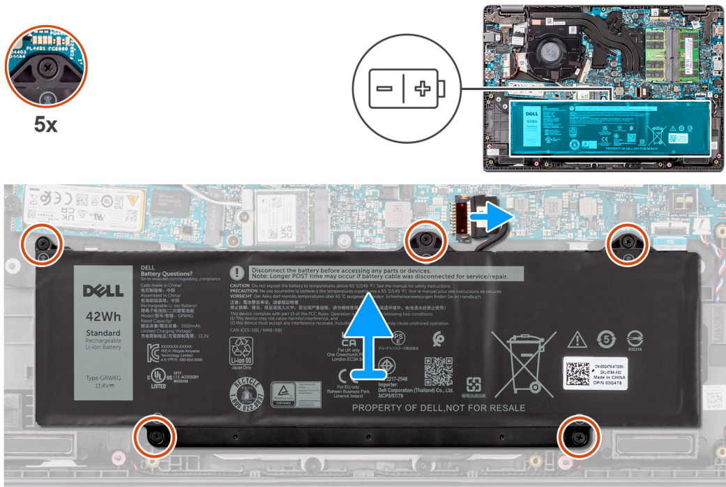
Ilustración 24. Extracción de la batería
