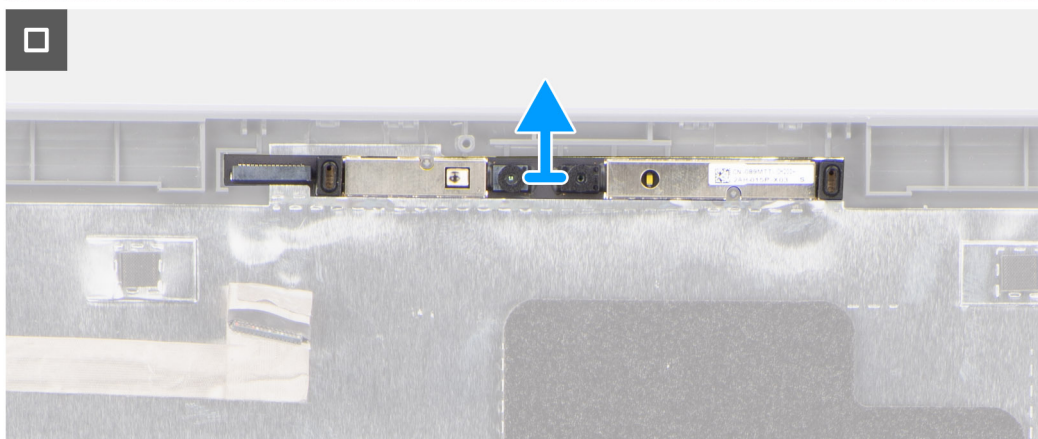
Ilustración 66. Extracción de la cámara
