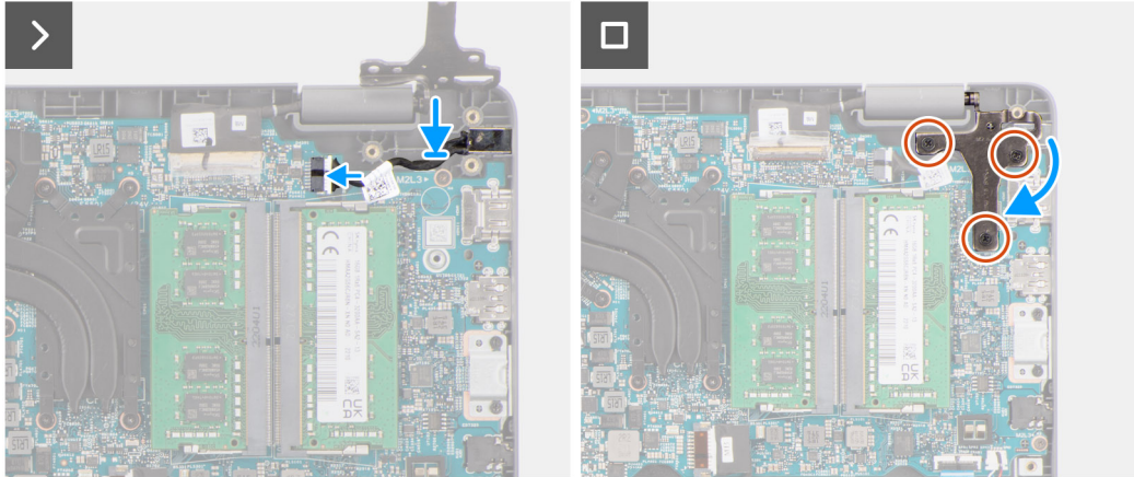
Ilustración 28. Instalación del puerto del adaptador de alimentación
