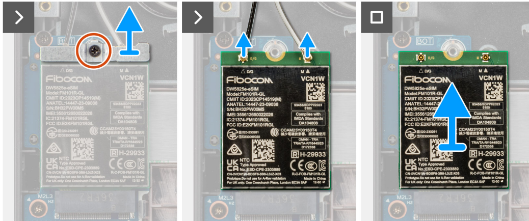
Ilustración 16. Extracción de la tarjeta WWAN
