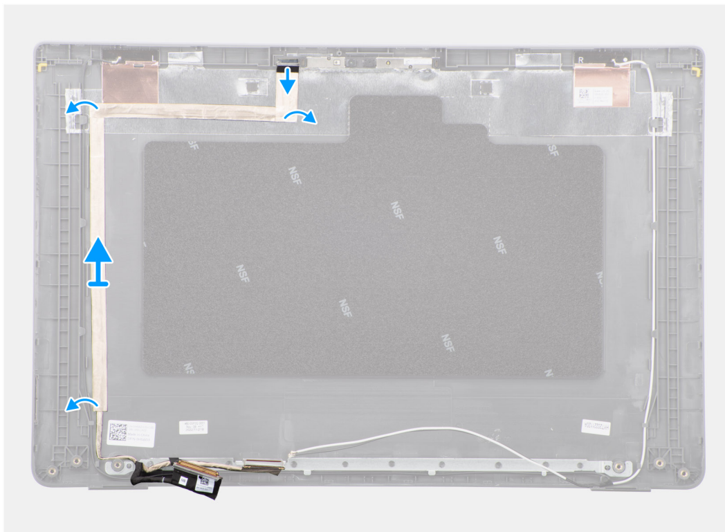
Ilustración 68. Extracción del cable de eDP
