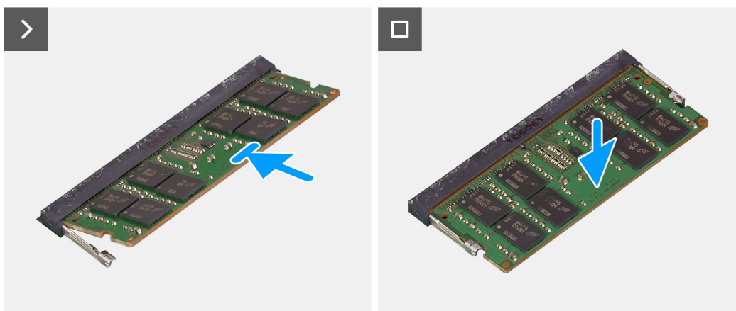
Ilustración 13. Instalación de los módulos de memoria
