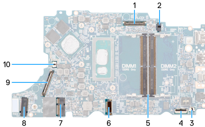
Ilustración 41. Conectores de la tarjeta madre: parte frontal
