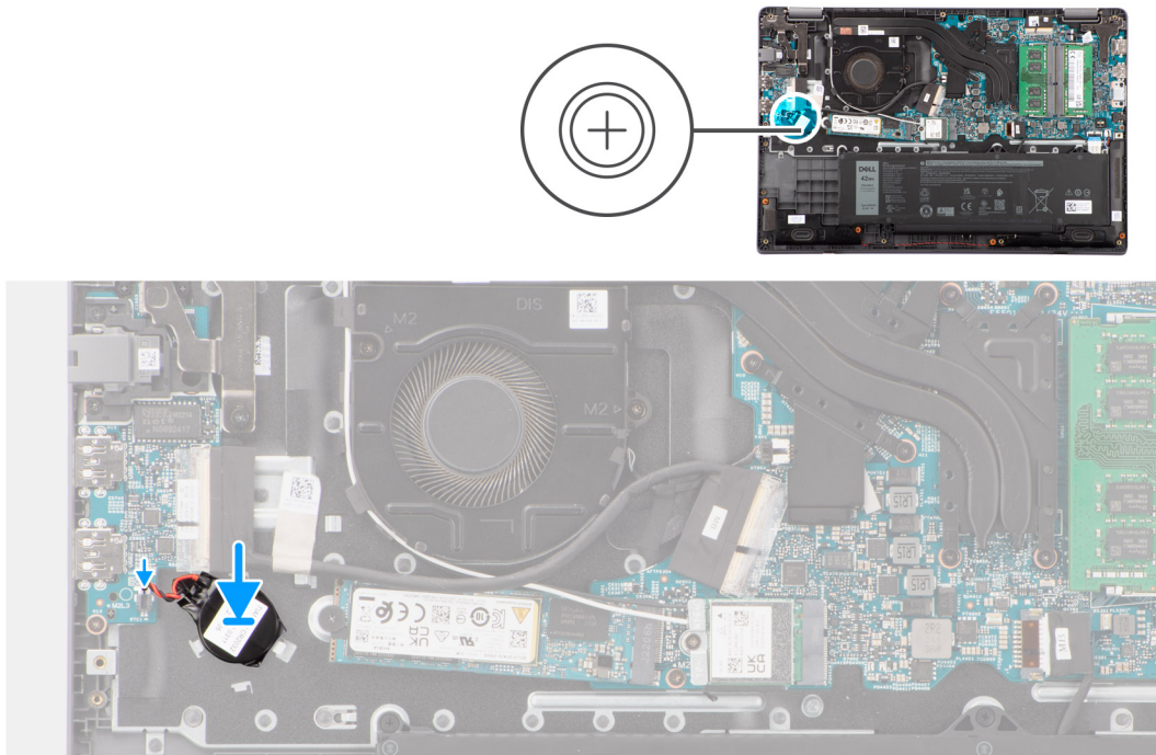
Ilustración 19. Instalación de la batería de tipo botón
