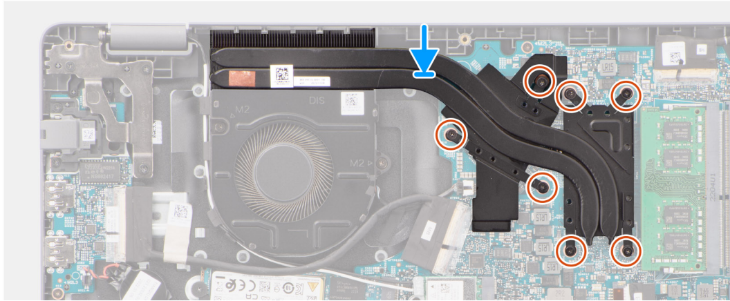
Ilustración 32. Instalación del disipador de calor para gráficos discretos
