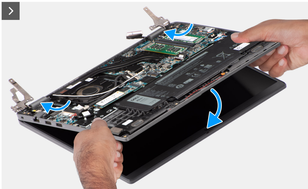
Ilustración 51. Instalación del ensamblaje de la pantalla
