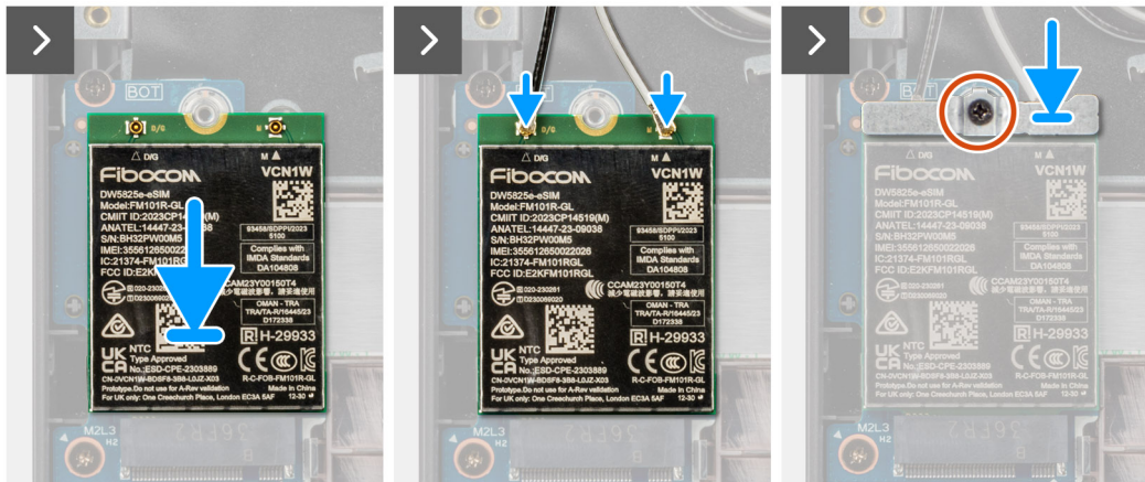
Ilustración 17. Instalación de la tarjeta WWAN
