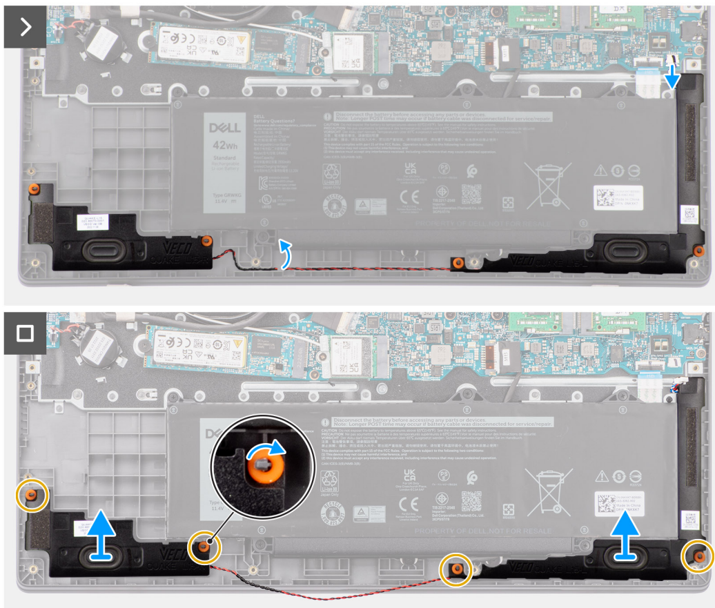
Ilustración 20. Extracción de los parlantes
