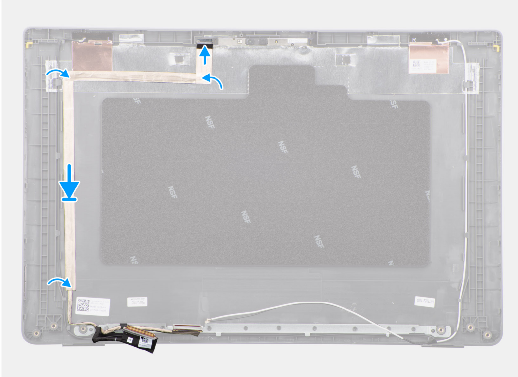
Ilustración 69. Instalación del cable eDP
